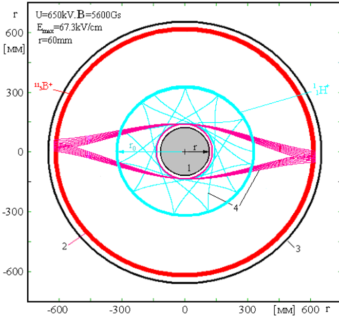
Рис. 13. Траектории движения (4) осциллирующих ионов водорода и ^{11}_5B^+ вблизи потенциального электрода с разными эмиттерами. В левом верхнем углу начальные условия при расчете. Для протона \varepsilon = 280 кэВ; для ^{11}_5B^+ \varepsilon = 629 кэВ, разность потенциалов между эмиттерами – 220 кВ. 1 – потенциальный электрод r_0 = 60 мм, 2 – эмиттер ^{11}_5B^+ , 3 – вакуумная камера 4 – траектории движения ионов.
