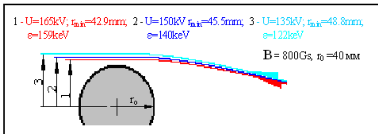
Рис. 8. Траектории движения {}^2_1\text{D}^+ при разных напряжениях на потенциальном электроде.
