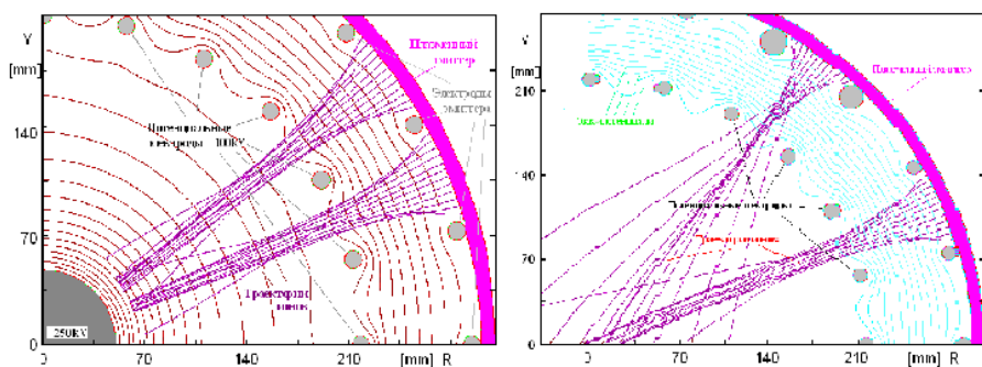
Рис. 17. Распределение электрического поля и траектории ионов в системе с дополнительными потенциальными электродами и разными электродами в эмиттере без магнитного поля (с центральным потенциальным электродом и без). Эквипотенциалы – через 10 кВ.
