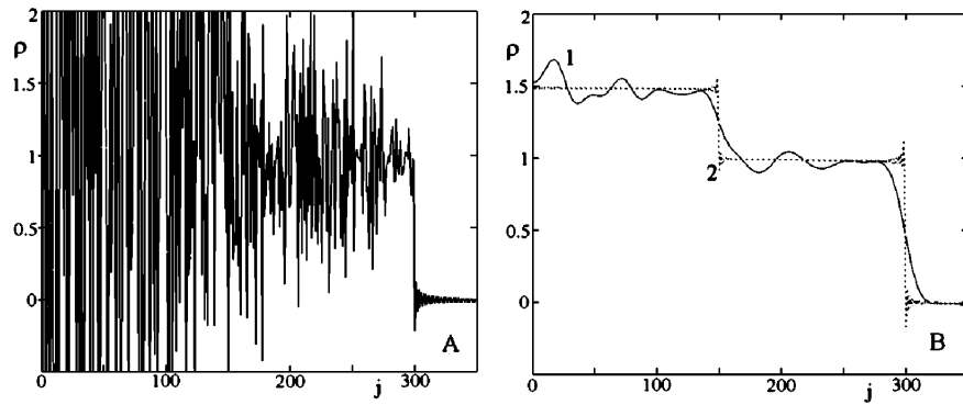
Рис. 6: А – прямое восстановление методом интегральных преобразований радиального распределения плотности при наличии шума. В – восстановление при наличии шума, но с фильтрацией (график 1), и прямое восстановления в отсутствии шума (график 2). Здесь: \rho – плотность ( \text{г/см}^3 ), j – номер слоя.
