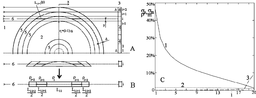
Рис. 5: А – Условная схема томографии аксиально-симметричного объекта: 1 – пучок СИ, 2 – исследуемый объект (заряд), 3 – многоэлементный детектор, 4 – чувствительные элементы (шириной \Delta ), 5 – concentрические слои (также шириной \Delta ), 6 – луч, приходящий от источника СИ на данный участок элемента; y – расстояние от края элемента с номером i до луча 6, а x – расстояние вдоль луча.
