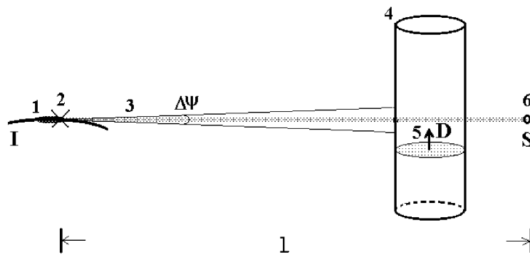
Рис. 1: Рассматриваемая схема теневой рентгенографии. Ступок (банч) 1 релятивистских электронов, двигаясь в магнитном поле, излучает по касательной к траектории синхротронное излучение. Из точки 2 ("источник") пучок 3 рентгеновской компоненты излучения (с углом раскрытия конуса \Psi ) попадает на исследуемый образец ("заряд") 4 с распространяющейся в нем со скоростью D ударной (детонационной) волной 5, и далее – на детектор 6 ( S – площадь детектора, l – расстояние до источника).
