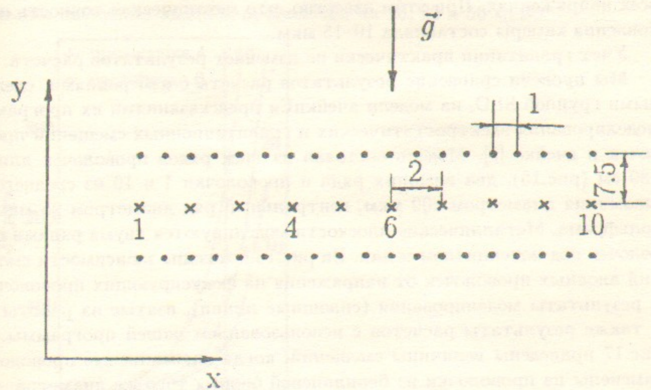
Рис.12. Модель пропорциональной камеры.
