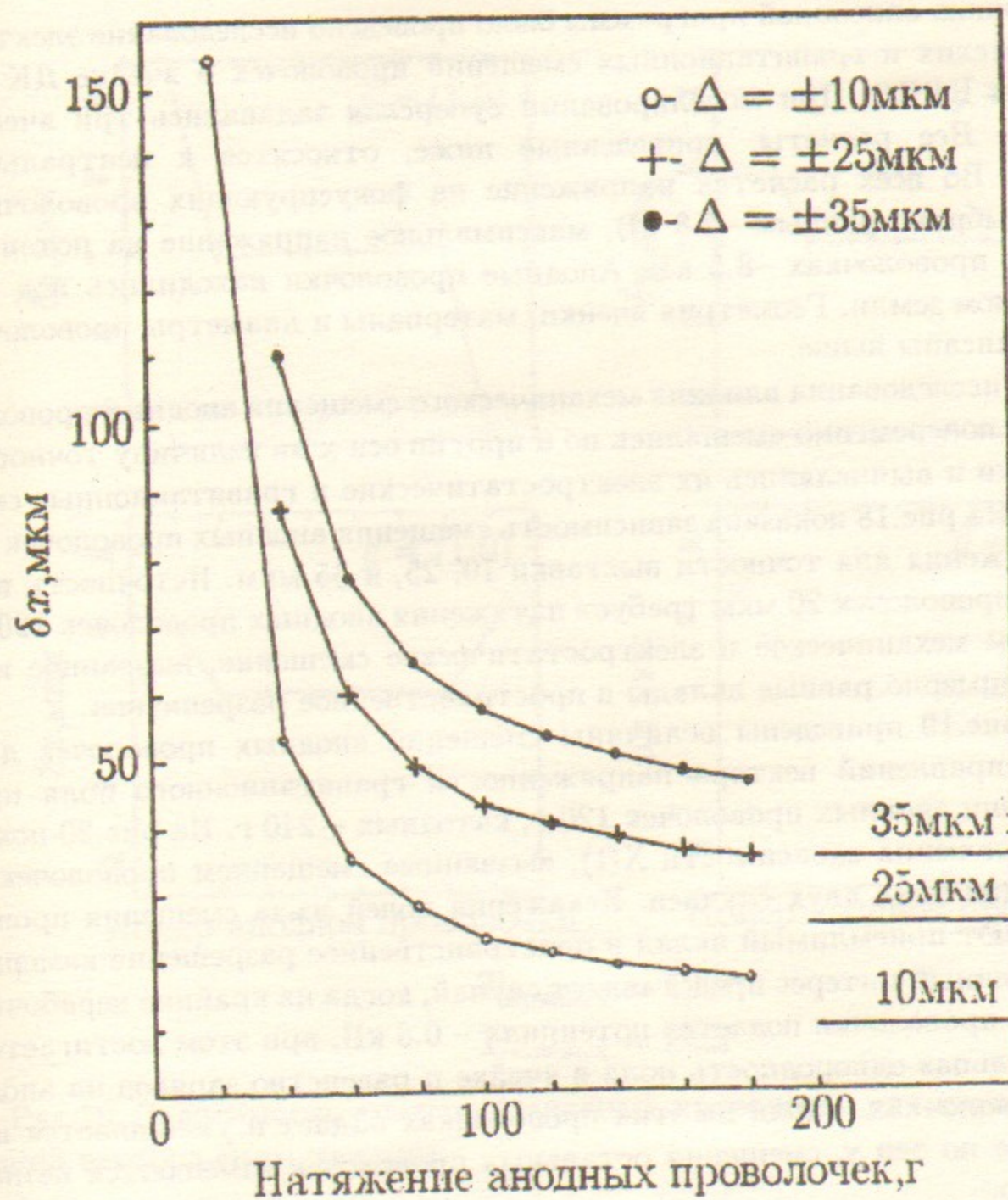
Рис.18. Зависимость смещений анодных проволочек от их натяжения для точности выставки проволочек 10, 20 и 50 мкм.
