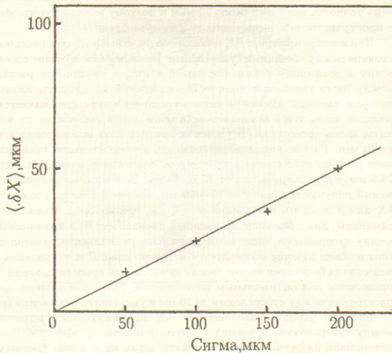
Рис.5. Среднее по ячейке искажение X(t) – зависимости как функция точности выставки полевых проволочек.
