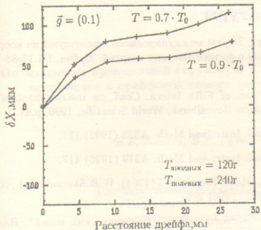
Рис.21. Искажения X(t) – зависимости из-за уменьшения натяжения проволочек в ячейке ДК до 90 и 70%.
