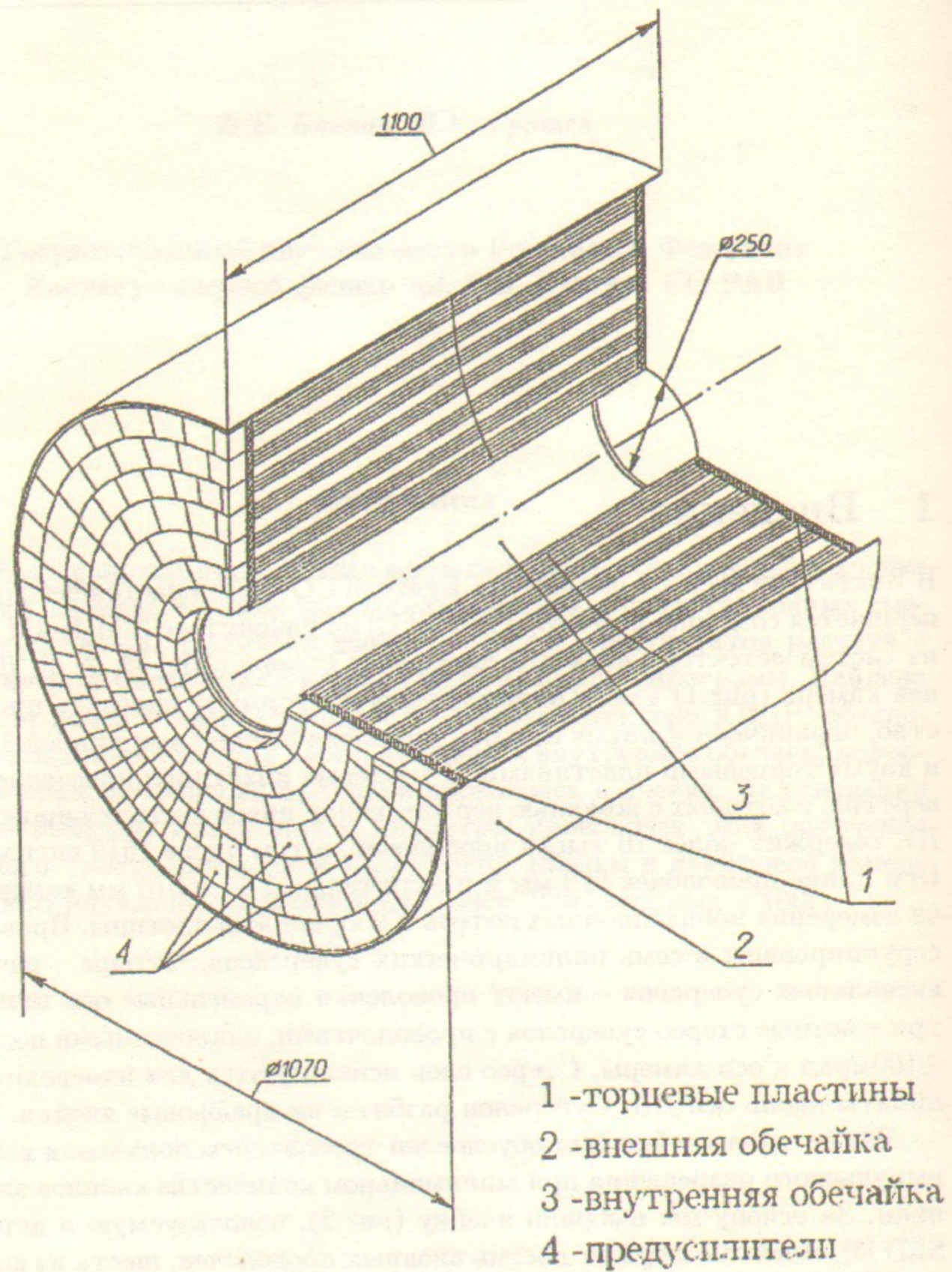
Рис.1. Общий вид дрейфовой камеры.
