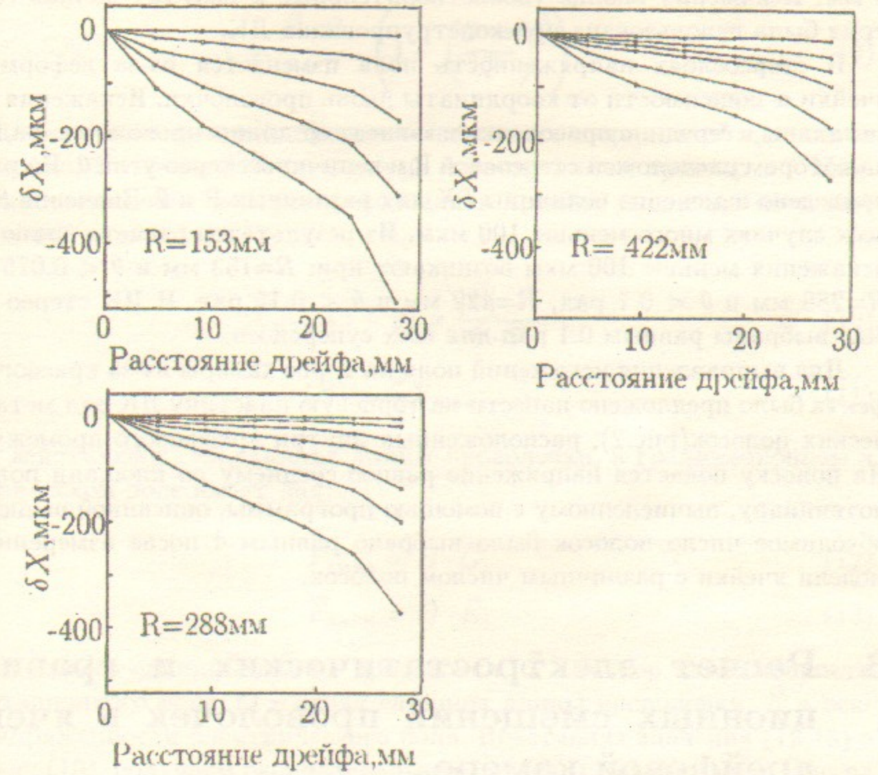
Рис.10. Искажения X(t) – зависимости от стереоугла для трех стереослоев, расположенных на расстояниях 153 мм, 288 мм и 422 мм. Стереоугол на графике изменяется от значения 25 мрад. с шагом 25 мрад.
