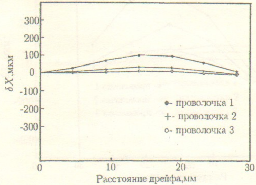
Рис.9. Искажения X(t) – зависимости для суперслоя от экрана под оптимальным потенциалом, расположенного на расстоянии 5 мм от него.
