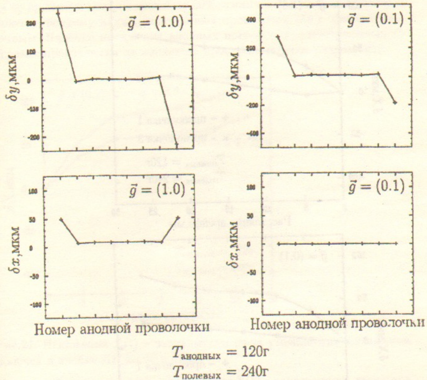
Рис.19. Зависимость смещений анодных проволочек для двух направлений вектора силы тяжести.
