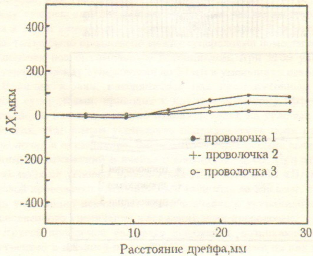
Рис.7. Искажения X(t) – зависимости для суперслоям с экраном на расстоянии 10 мм под оптимальным потенциалом.
