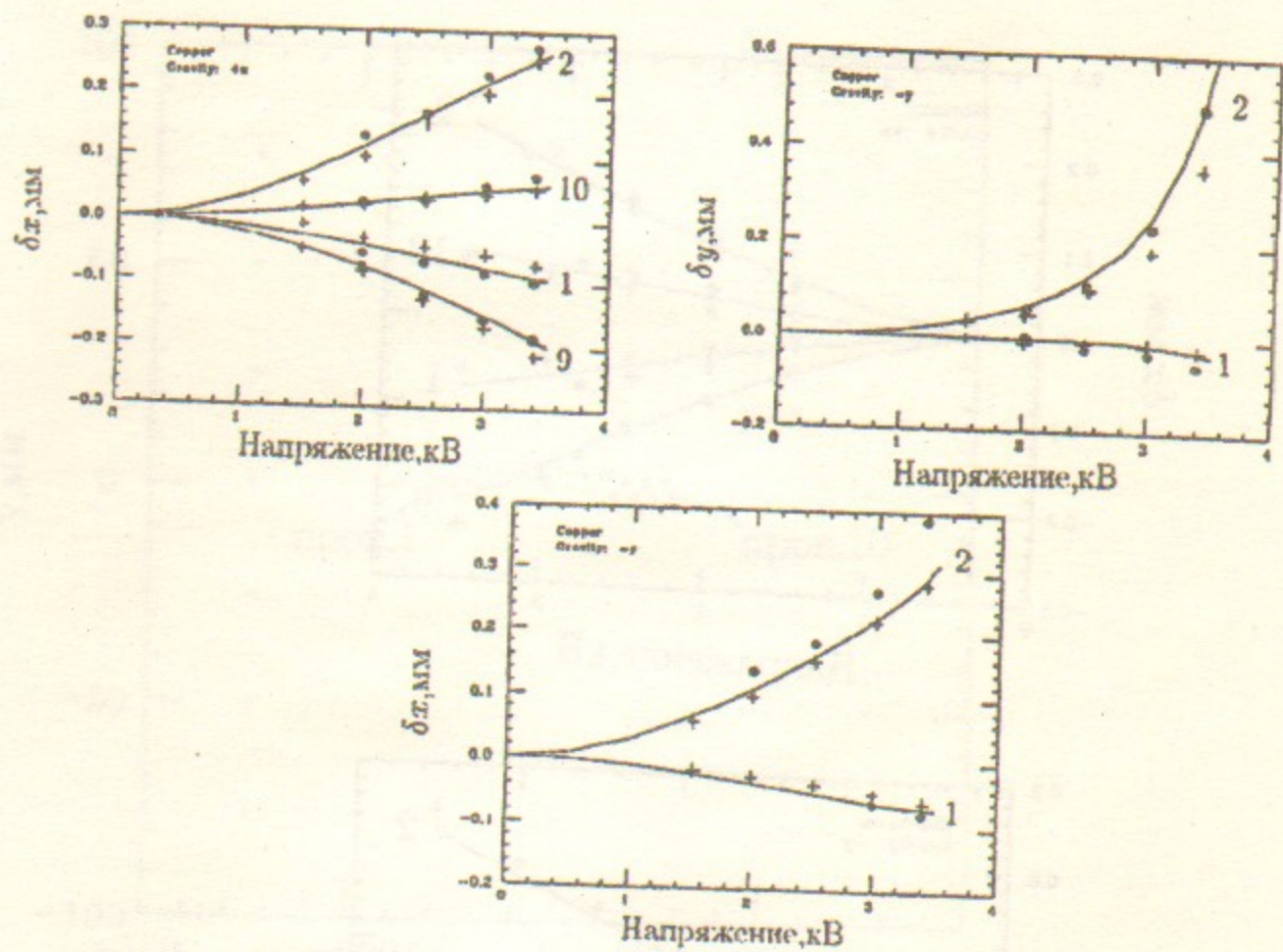
Рис.17. Зависимость смещений анодных проволочек от напряжения на фокусирующих проволочках для двух направлений вектора силы тяжести.
