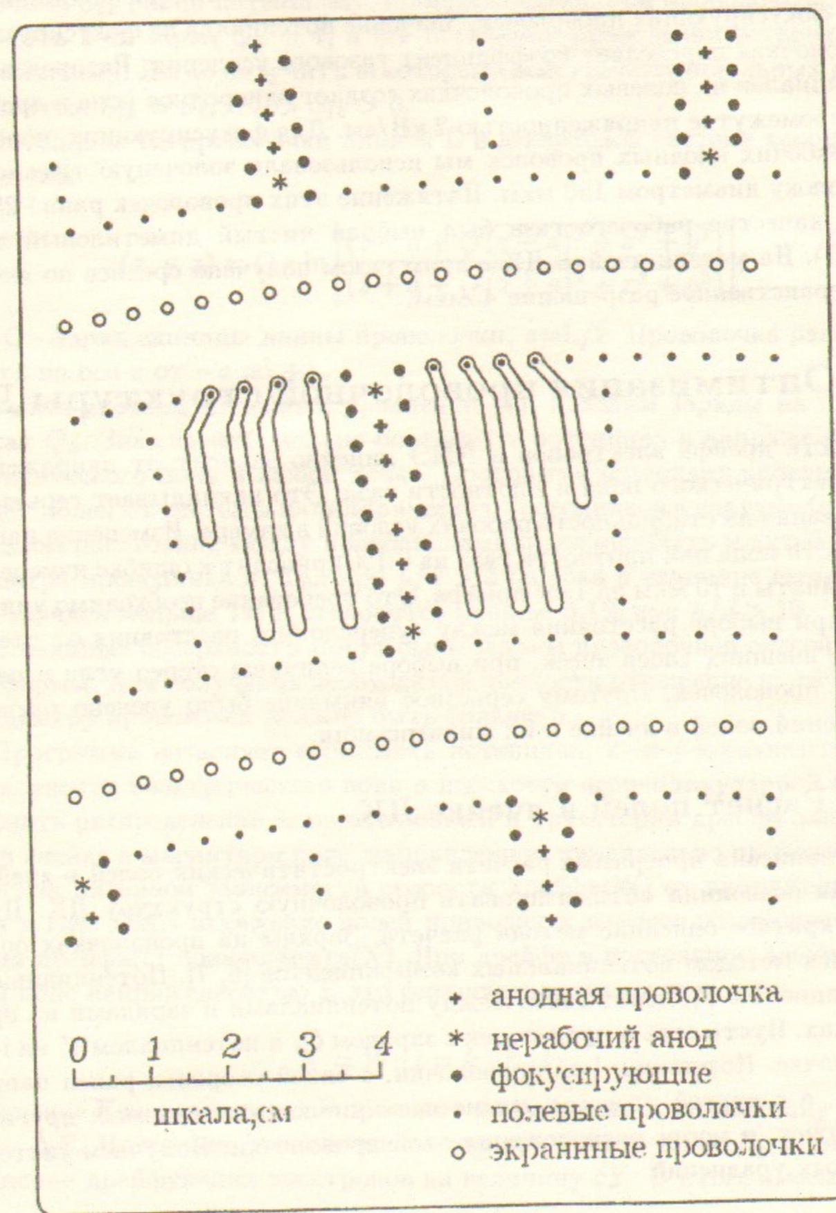
Рис.2. Ячейка дрейфовой камеры.
