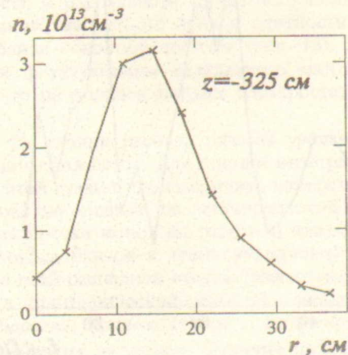
Рис.16. Радиальный профиль плотности плазмы в транспортирующей области для z = -325 см
