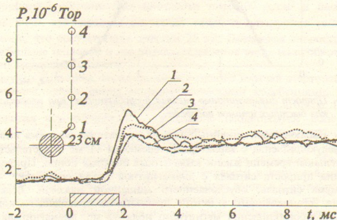
Рис.22. Зависимости давления водорода в пробкотроне от времени
