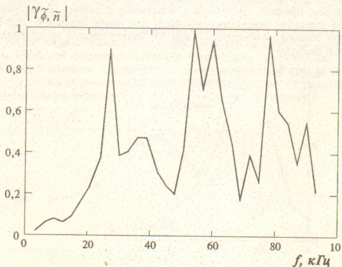
Рис. 17. Спектр когерентности флуктуаций плотности и азимутального электрического поля во входной пробке
