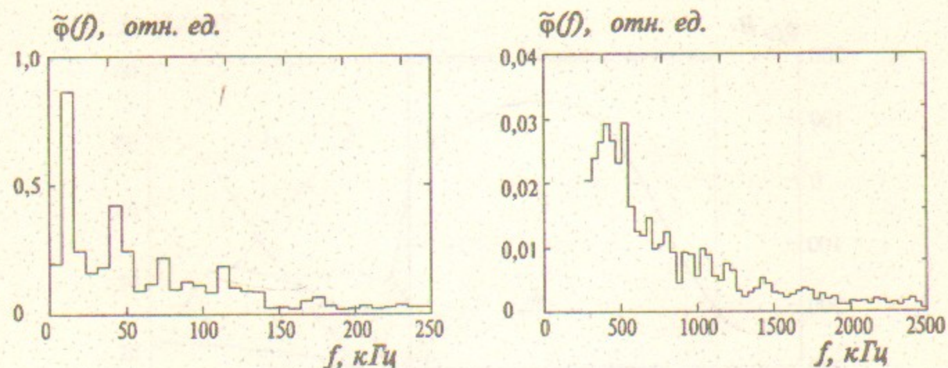
Рис.13. Спектр электростатических флуктуаций во входной пробке
