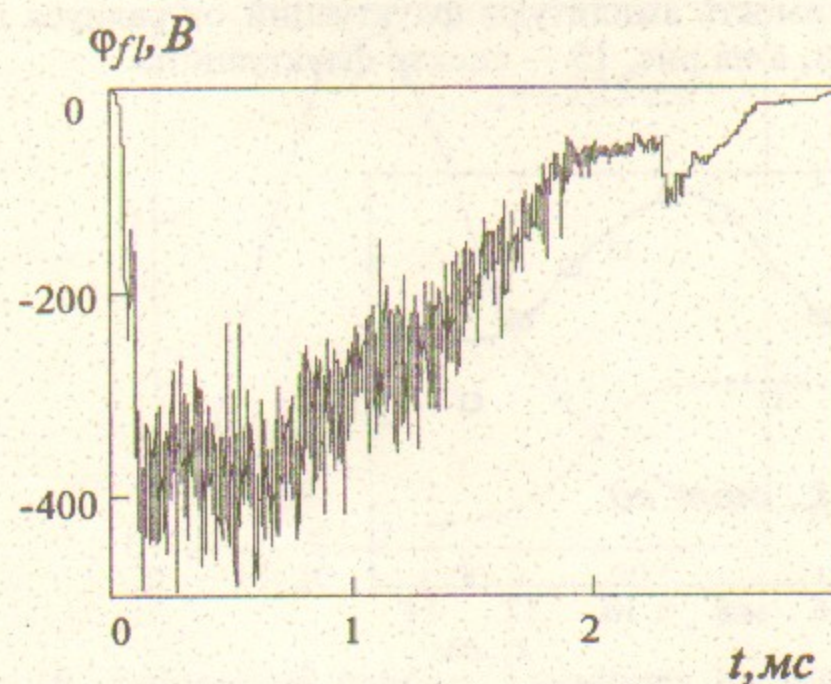
Рис.12. Осциллограмма плавающего потенциала зонда ( z=-115 см)
