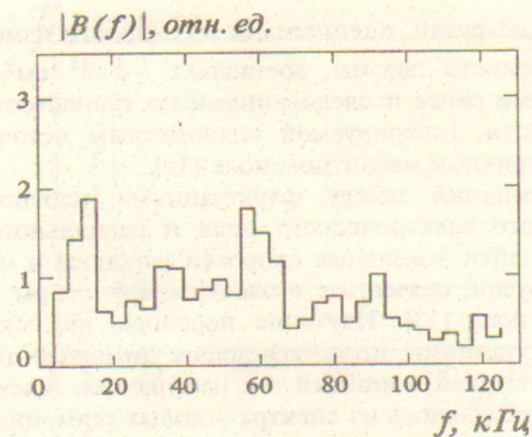
Рис.15. Спектр флуктуаций азимутального магнитного поля в транспортирующей области
