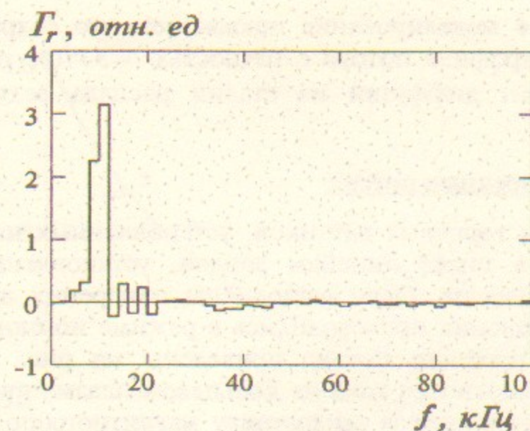
Рис. 18. Спектральная плотность потока частиц, вызванного магнитными флуктуациями в транспортирующей области
