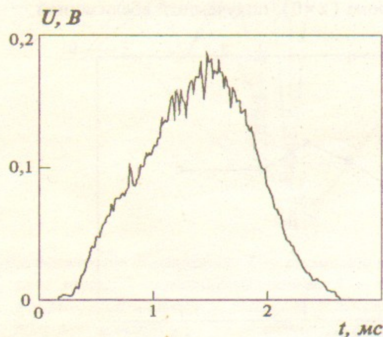
Рис.5. Осциллограмма диамагнетизма стартовой плазмы в пробкотроне ( z=25 см)
