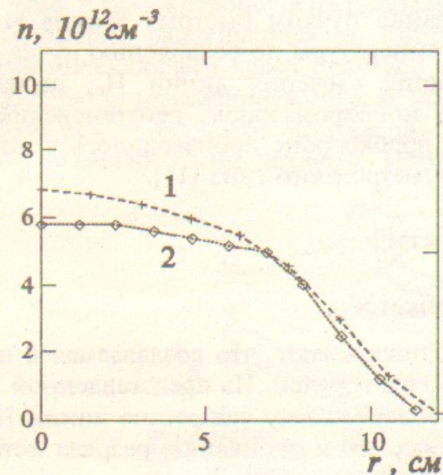
Рис.4. Радиальные профили плотности плазмы в пробкотроне. 1 — в центральной плоскости, 2 — в плоскости z=25 см
