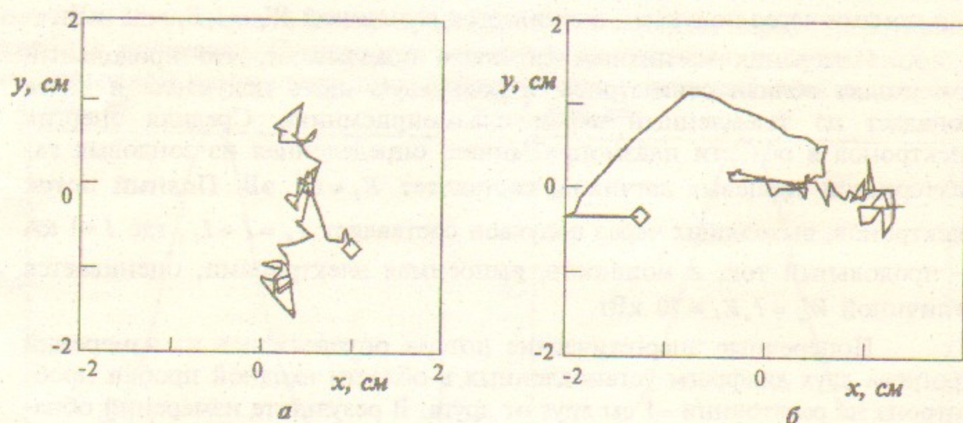
Рис.21. Перемещения центра плазменного шнура на стадии распада при включенном (а) и выключенном (б) полукаспе. Ромбы указывают начало движения
