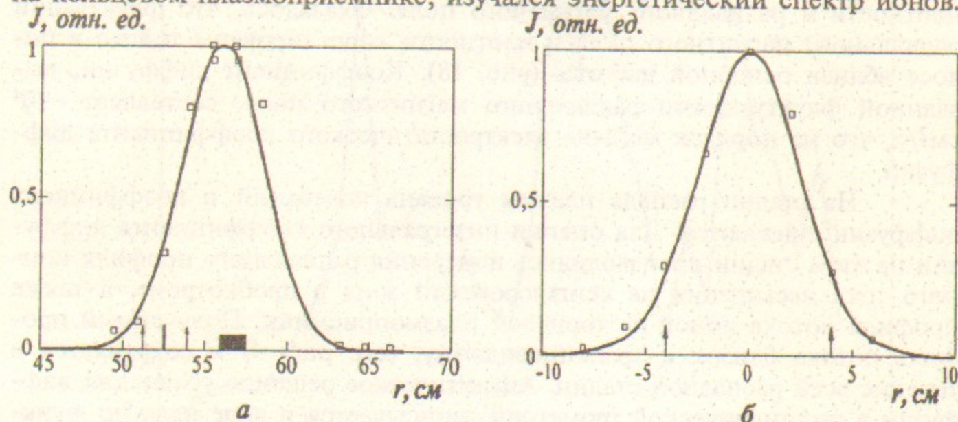
Рис.19. Измеренные профили потока плазмы на кольцевой плазмоприемник полукаспа (а) и через осевую пробку (б). Стрелками указаны границы зоны адиабатичности. Положение сепаратрисы отмечено чертой, проекция газоразрядного канала показана прямоугольником
