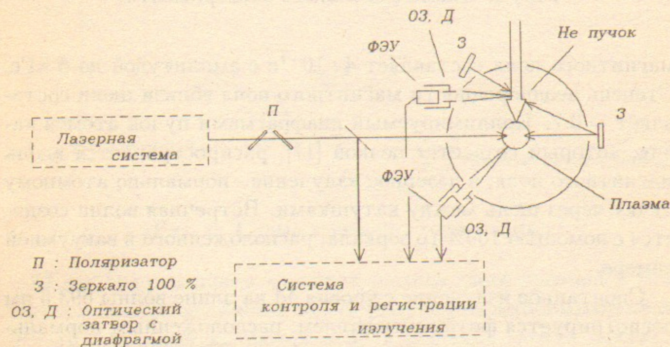
Рис. 3: Схема измерения магнитного поля в плазме.
