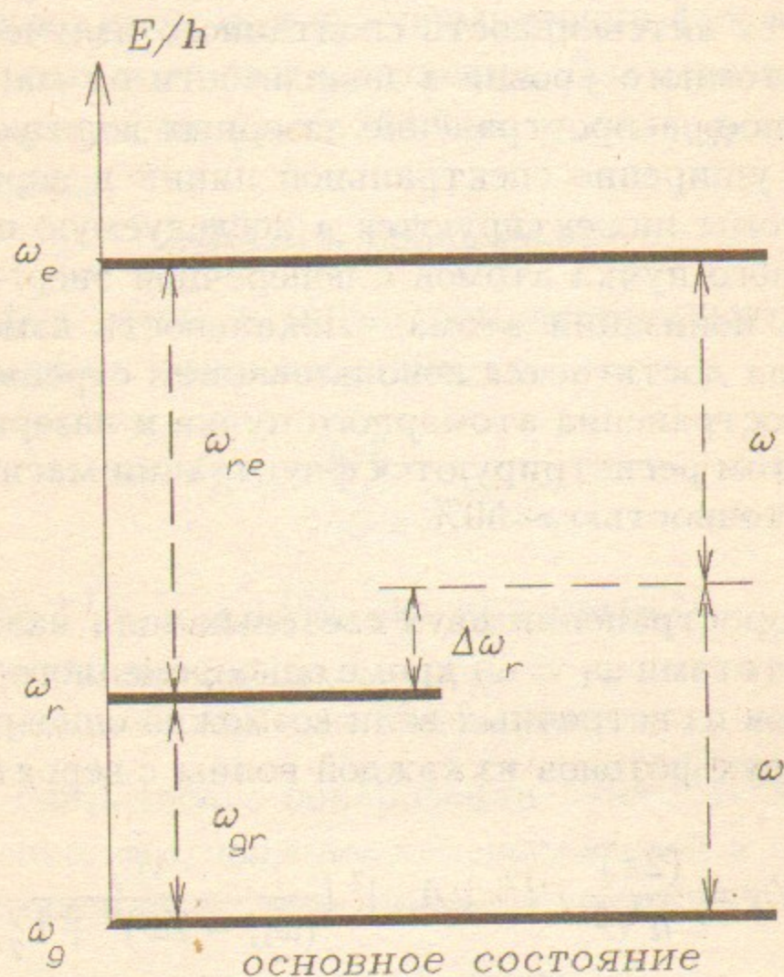
Рис. 1: Двухфотонный переход в трехуровневой системе.
