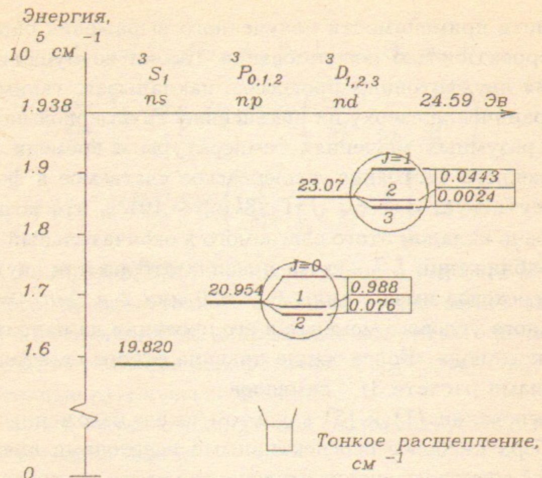
Рис. 2: Схема уровней в атоме гелия.
