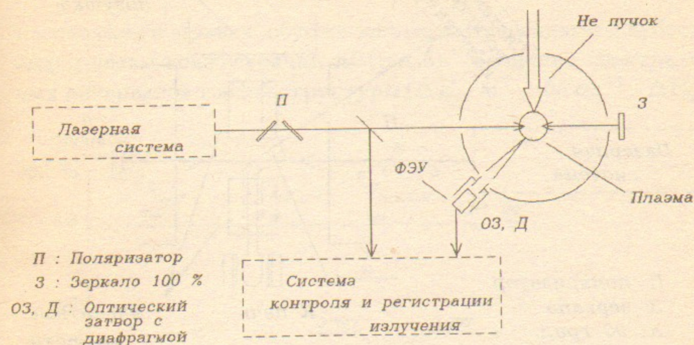
Рис. 3: Схема измерения магнитного поля в плазме.
