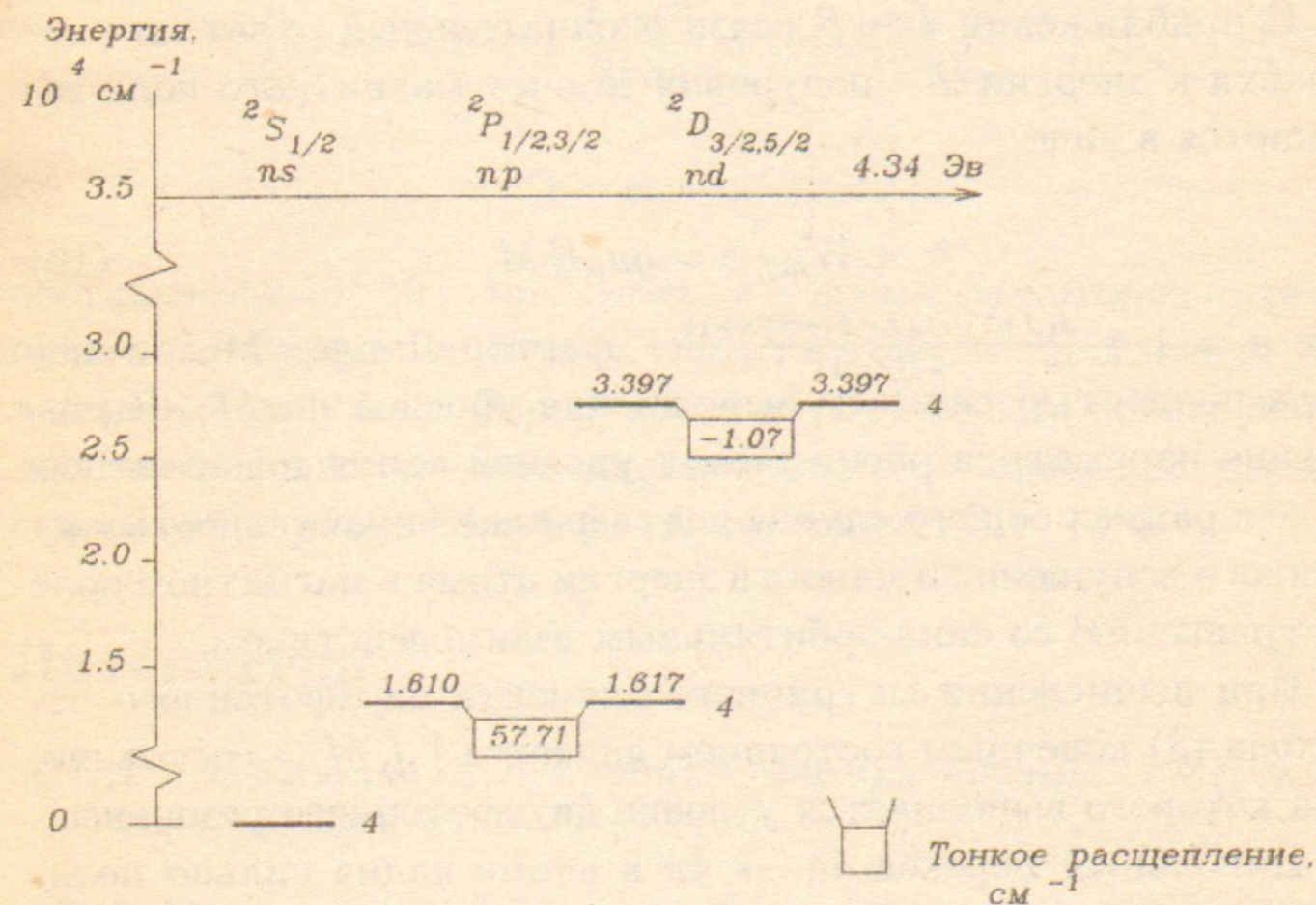
Рис. 6: Схема уровней атома калия.
