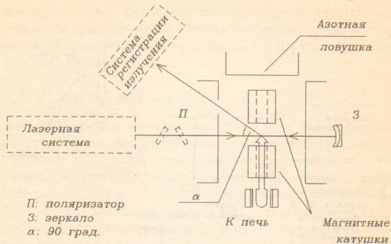
Рис. 5: Схема модельного эксперимента.
