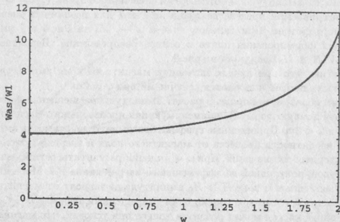
Рис.8 Зависимость вероятности W_{as} \equiv W(H \gg H_0) от энергии начального фотона ( w = \omega/m ).
