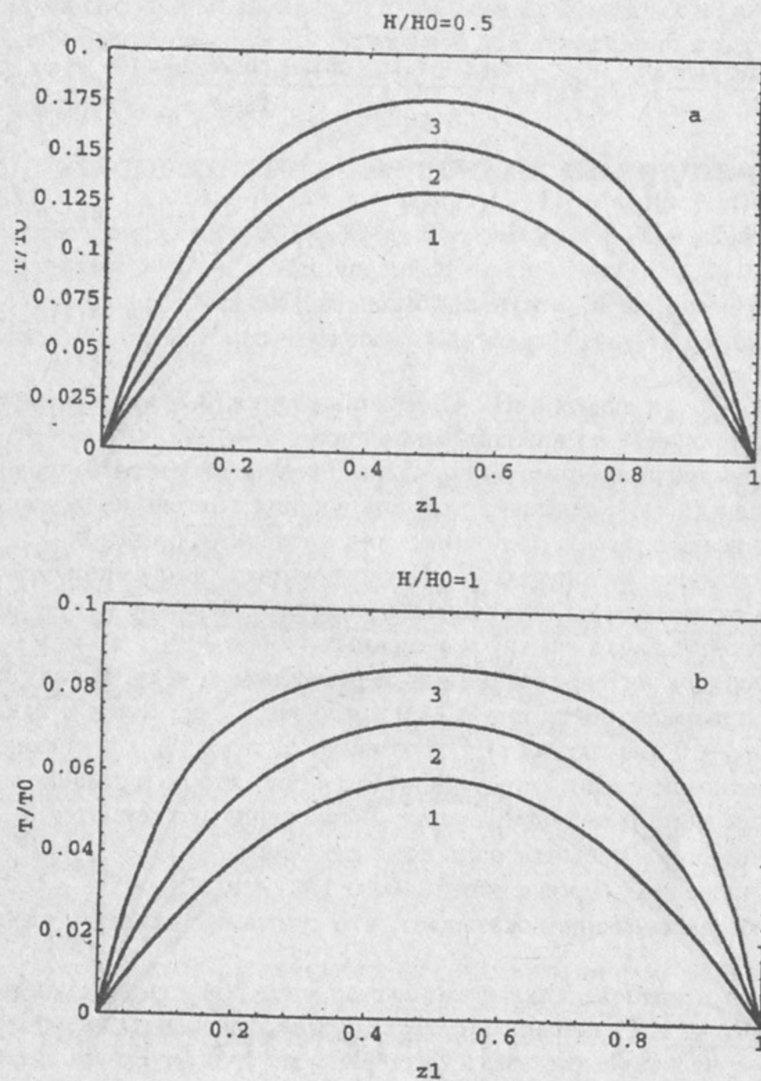
Рис.4 Зависимость амплитуды расщепления фотона от энергии одного из конечных фотонов ( z_1 = \omega_1/\omega ) для H = H_0/2 (рисунок а) и H = H_0 (рисунок б) для разных энергий начального фотона: \omega/m = 0.1 (1), \omega/m = 1.5 (2) и \omega/m = 1.9 (3). Амплитуда T нормирована на амплитуду T_0 , формула (3.4).
