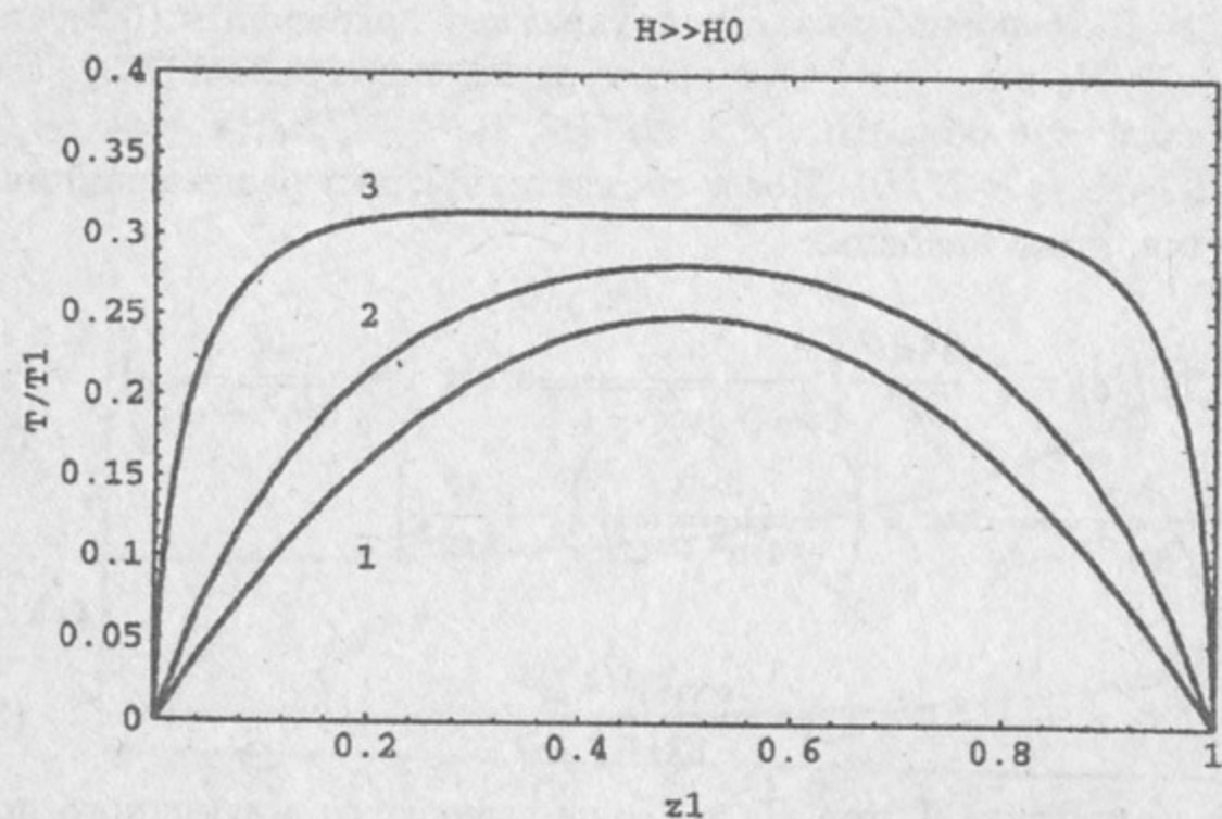
Рис.7 Зависимость амплитуды T от энергии конечного фотона для поля H \gg H_0 при разных энергиях начального фотона: \omega/m = 0.1(1) , \omega/m = 1.5(2) and \omega/m = 1.99(3) .
