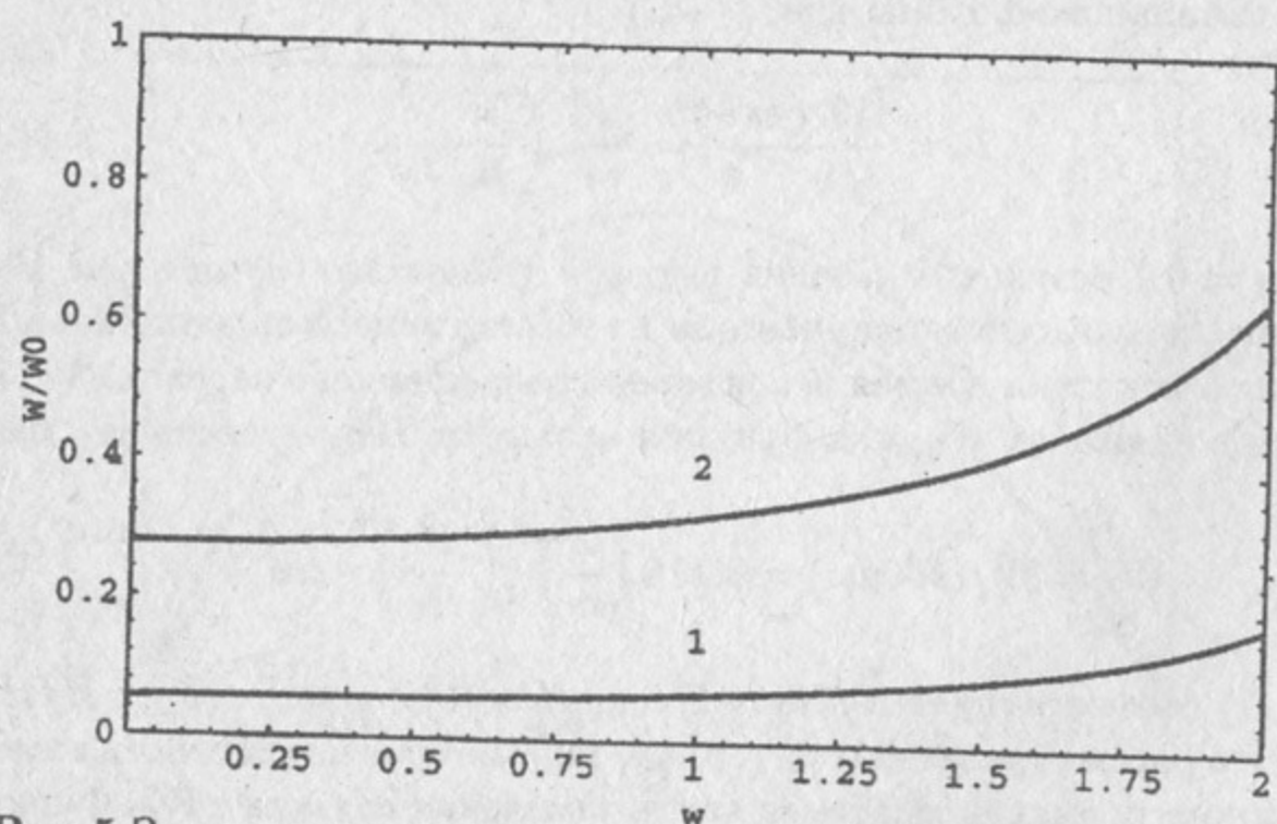
Рис.5 Зависимость полной вероятности расщепления фотона W (выраженной через вероятность W_0 , формула (3.5)) от энергии фотона ( w = \omega/m ) для H = H_0 (кривая 1) и H = H_0/2 (кривая 2).
