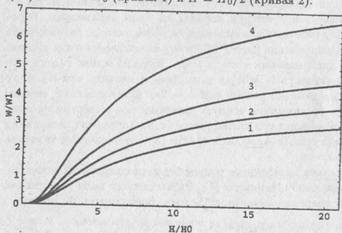
Рис.6 Зависимость полной вероятности расщепления фотона W (выраженной через вероятность W_1 , формула (3.6)) от магнитного поля (в единицах H_0 ) для разных энергий начального фотона: кривая 1 для w = \omega/m = 0.1 (эта кривая с хорошей точностью совпадает с вероятностью найденной с использованием эффективного лагранжиана ГЭ); кривая 2 для w = 1.1 ; кривая 3 для w = 1.5 ; кривая 4 для w = 1.9 .
