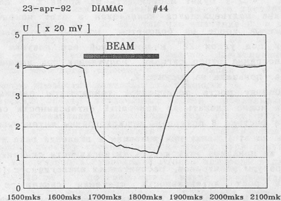
Рис. 6. Диамагнитный сигнал при работе пучков.
