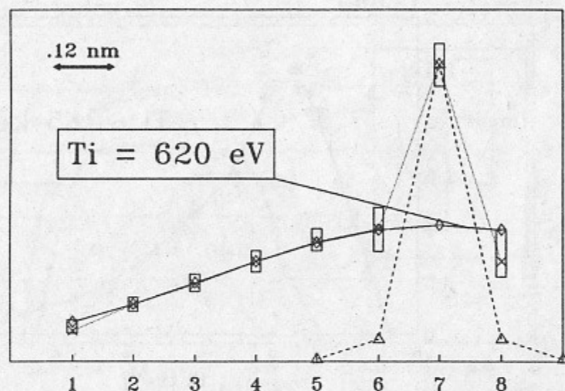
Рис.5. Доплеровские измерения ионной температуры.
