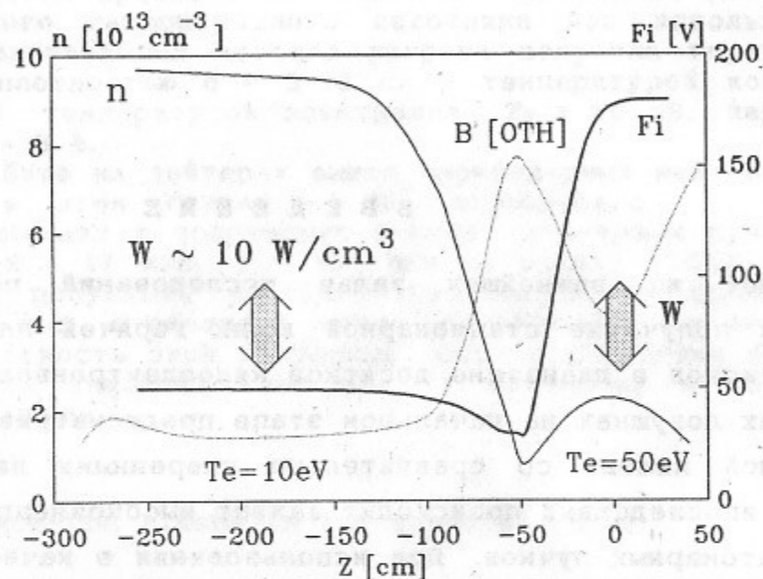
Рис. 1. Термобарьер, реализуемый на установке "Амбал-ЮМ"
