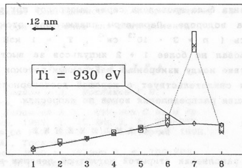
Рис. 11. Доплеровские измерения ионной температуры.
