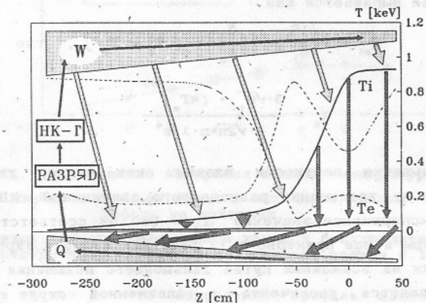
Рис.10. Диаграмма энергобаланса
