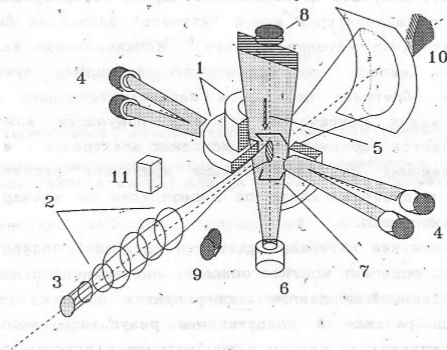
Рис. 2. Схема установки « АМБАЛ - ЮМ »
