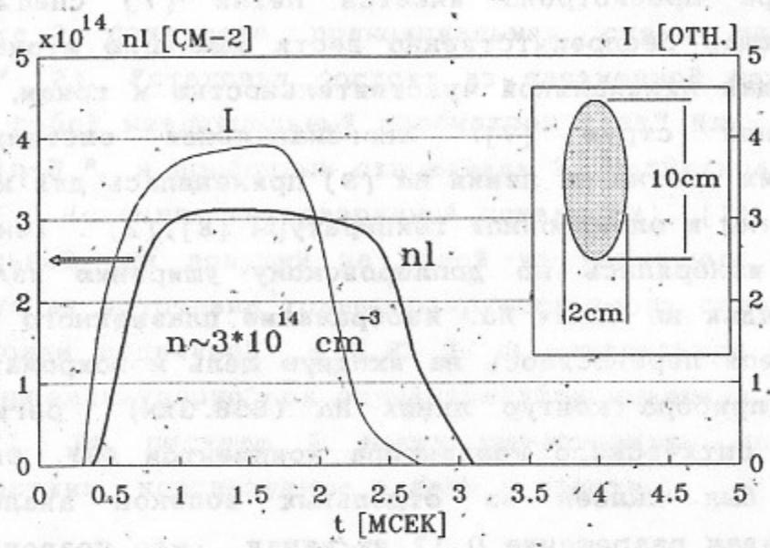
Рис. 3. Плотность плазмы в центре ловушки. Линейная плотность плазмы; ток дугового разряда источника; сечение плазмы в медианной плоскости (на уровне 1/2)
