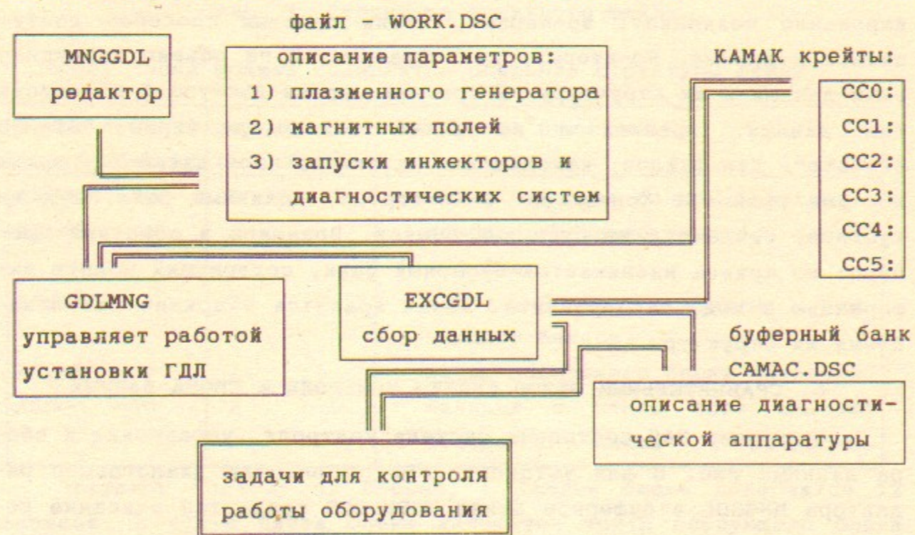
Рис.8. Схема управления и сбора данных установки ГДЛ.
