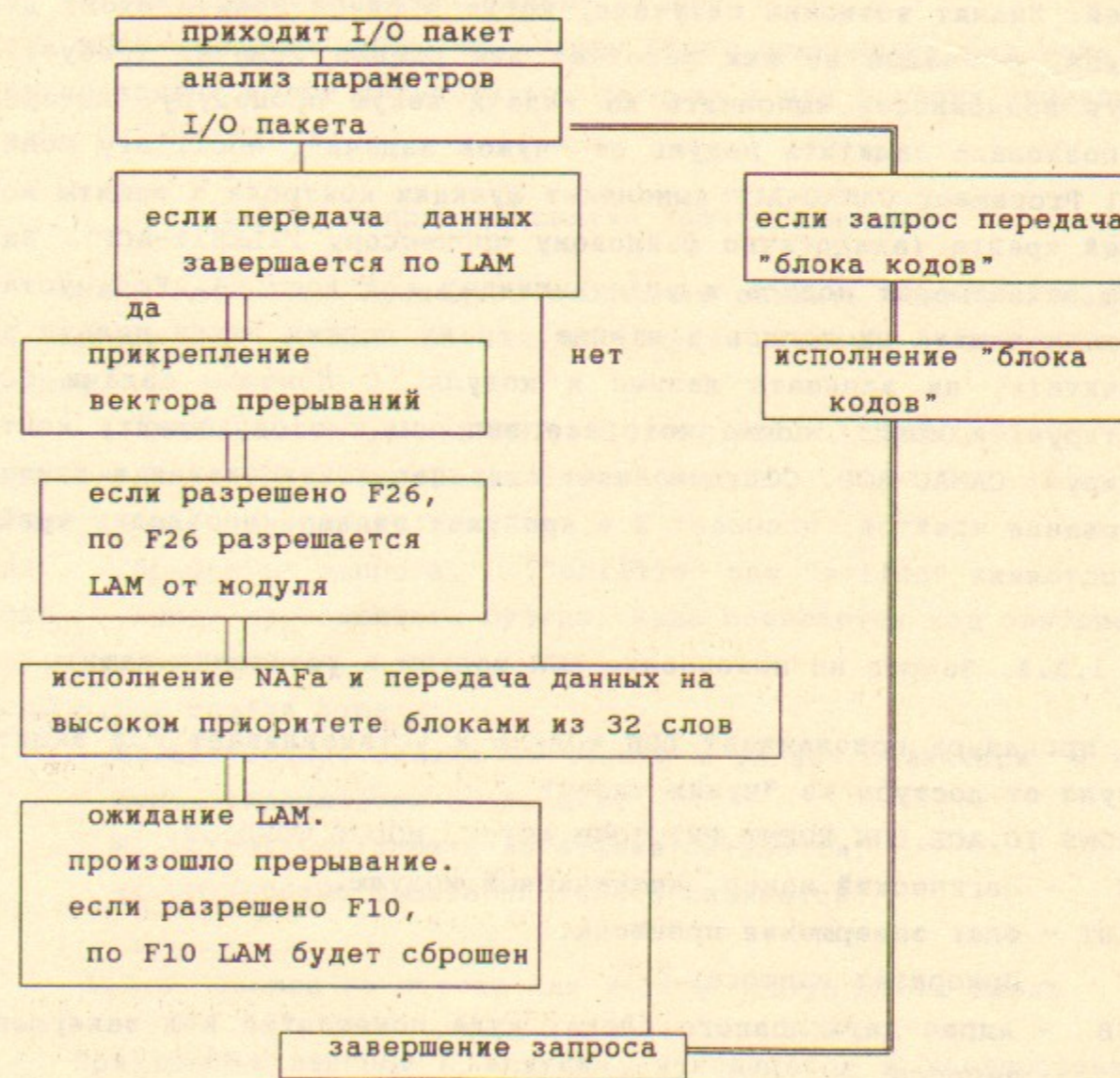
Рис. 4. Блок-схема КАМАК драйвера CCDRV: первому - CC0:, второму - CC1, и т.д. [4].
