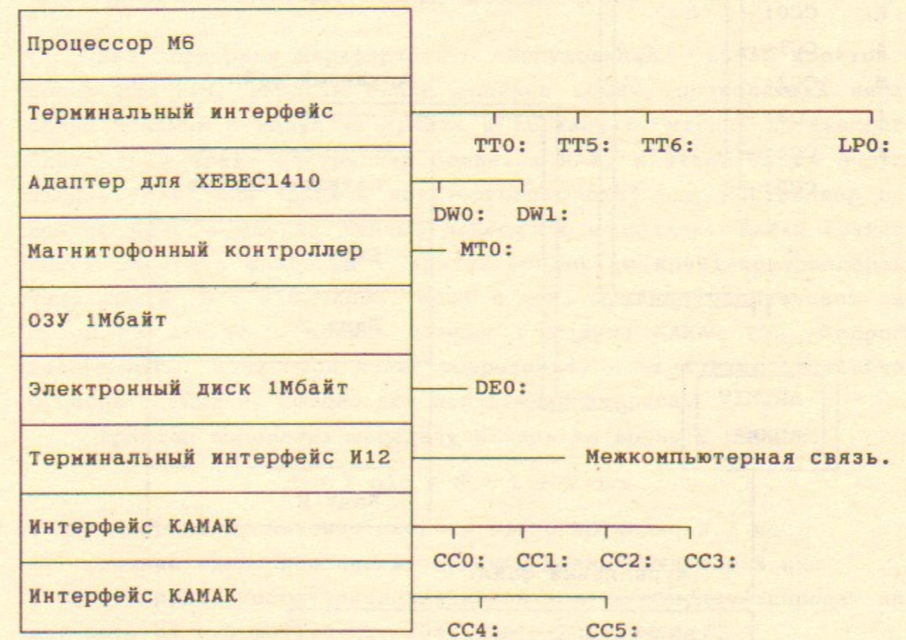
Рис. 2. Конфигурация "Электроники MC1212".
