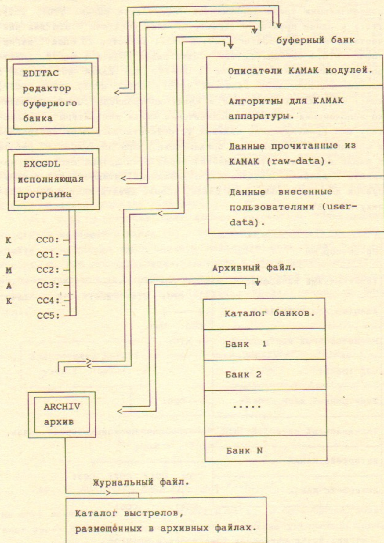
Рис. 3. Логическая схема DAS.
