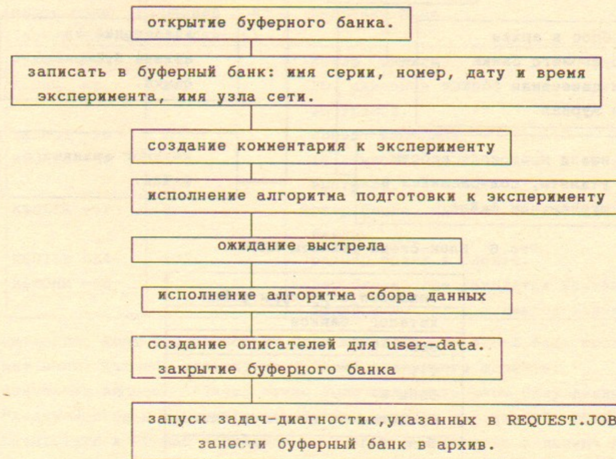
Рис. 5. Блок-схема управляющей утилиты EXCGDL.
