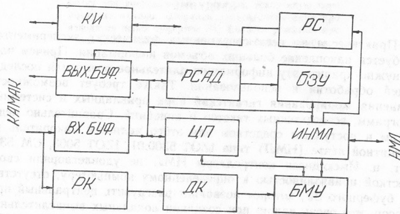
Рис. 1. Блок-схема контроллера.
