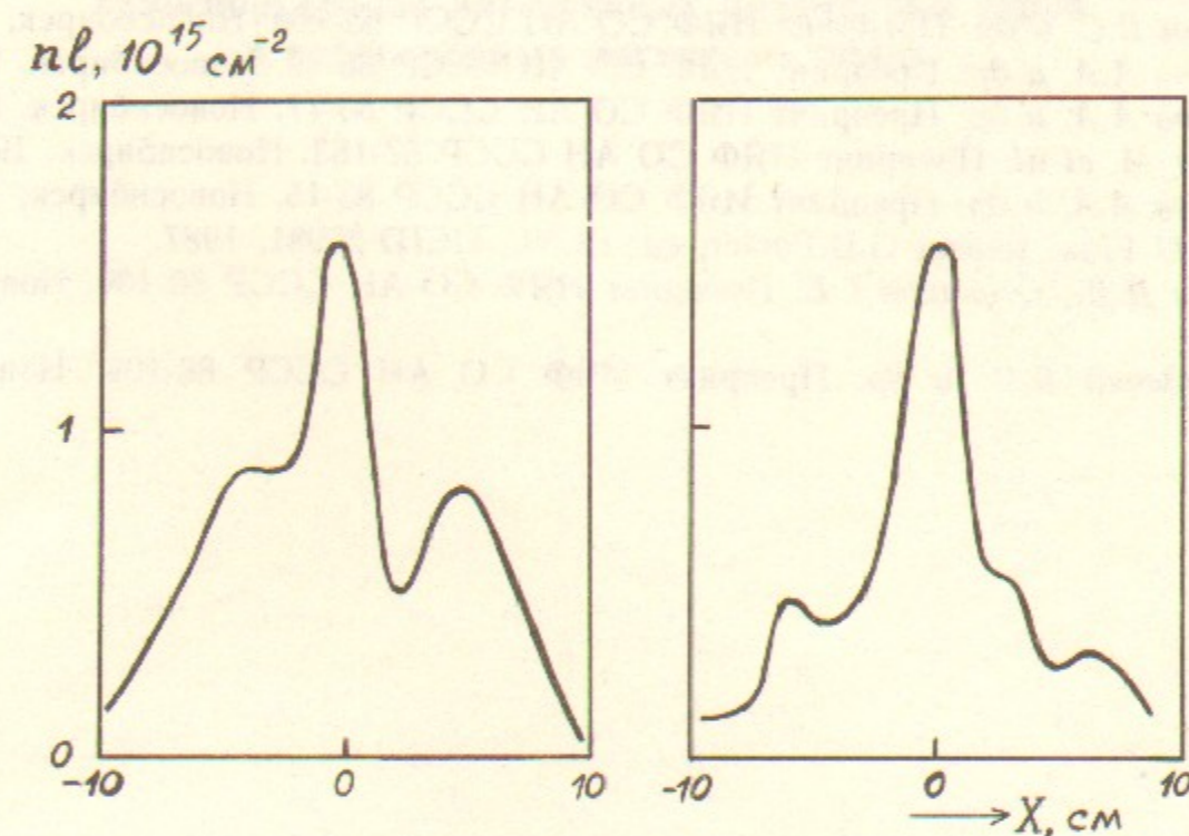
Рис. 30. Горизонтальный профиль линейной плотности плазменных струй при совместной работе пушек: а — при согласованном включении соленоида пушек; б — при согласованном включении соленоида щелевой пушки и при отключенных соленоидах кольцевых пушек.
