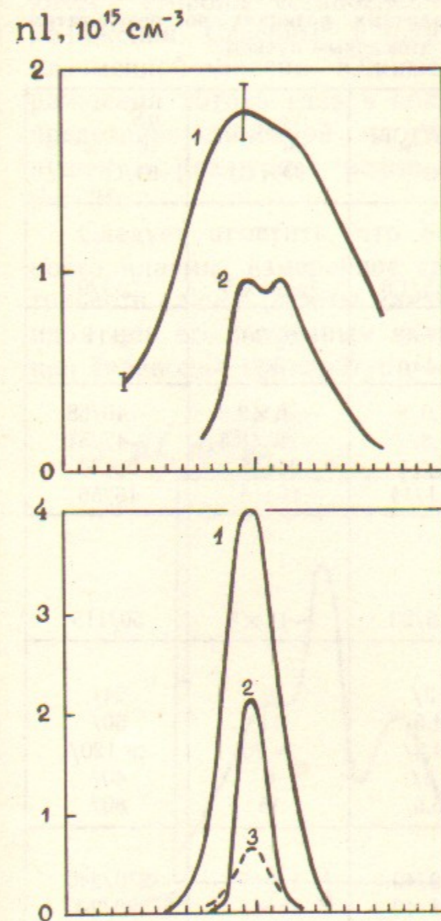
Рис. 27. Горизонтальный профиль линейной плотности плазменной струи щелевой пушки, установленной в центральном фланце торцевого бака: a —южного, b —северного; 1—согласованное включение соленоида пушки, 2—соленоид выключен, 3—встречное включение.
