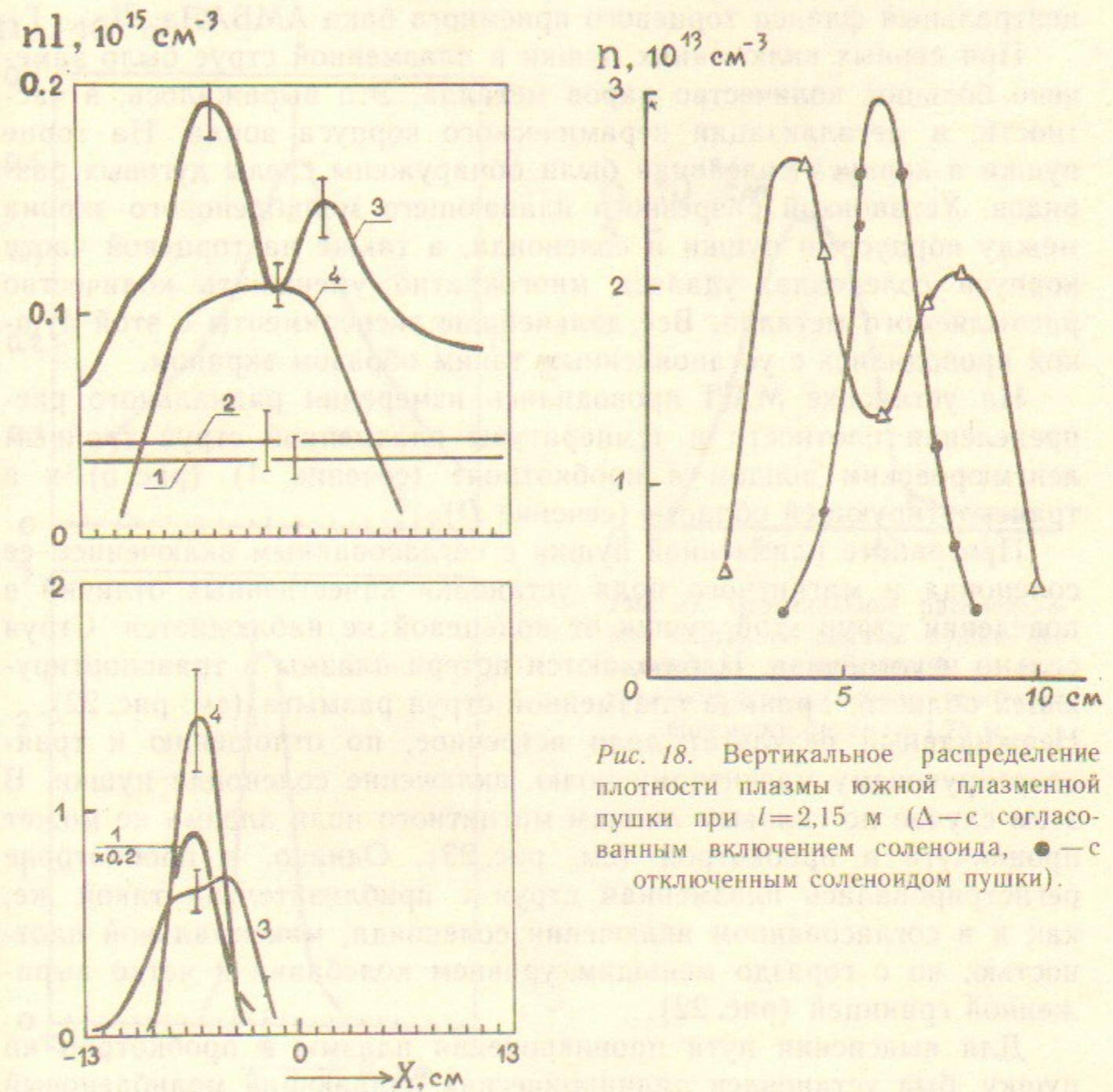
Рис. 17. Горизонтальный профиль линейной плотности плазменной струи: а — южной плазменной пушки; б — северной плазменной пушки: l=2,95 м (1); l=2,65 м (2); l=2,15 м (3, 4). 1, 2, 3 — согласованное включение соленоида пушки, 4 — соленоид пушки отключен.
