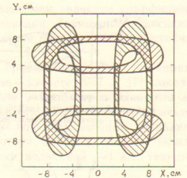
Рис. 3. Расчетная форма сечения струй мишенной плазмы в центральной плоскости пробкотрона.
