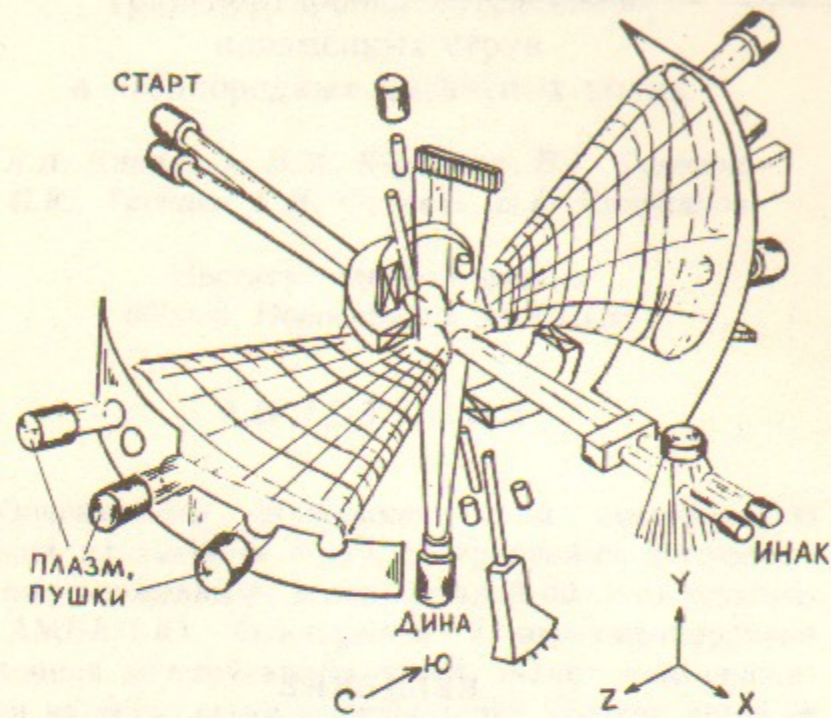
Рис. 1. Установка АМБАЛ-Ю.
