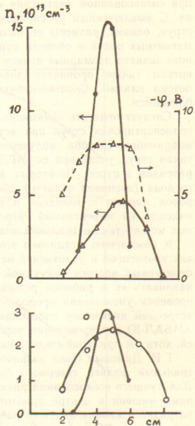
Рис. 26. Вертикальное распределение плотности плазмы n и потенциала \varphi осевой пушки, установленной в центральном фланце южного торцевого бака: a-l=1,75 м, b-l=2,25 м; \circ —согласованное включение соленоида пушки, \bullet —соленоид выключен; \Delta —встречное включение.
