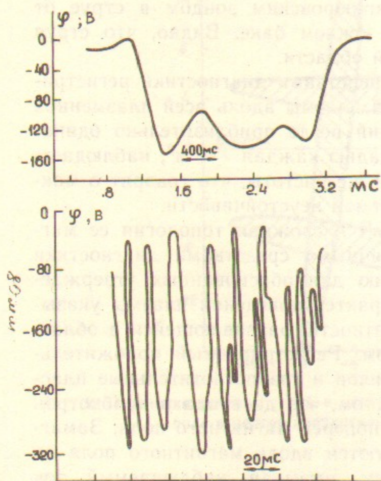
Рис. 10. Средняя величина и уровень колебаний потенциала плазмы \varphi в пробкотроне.
