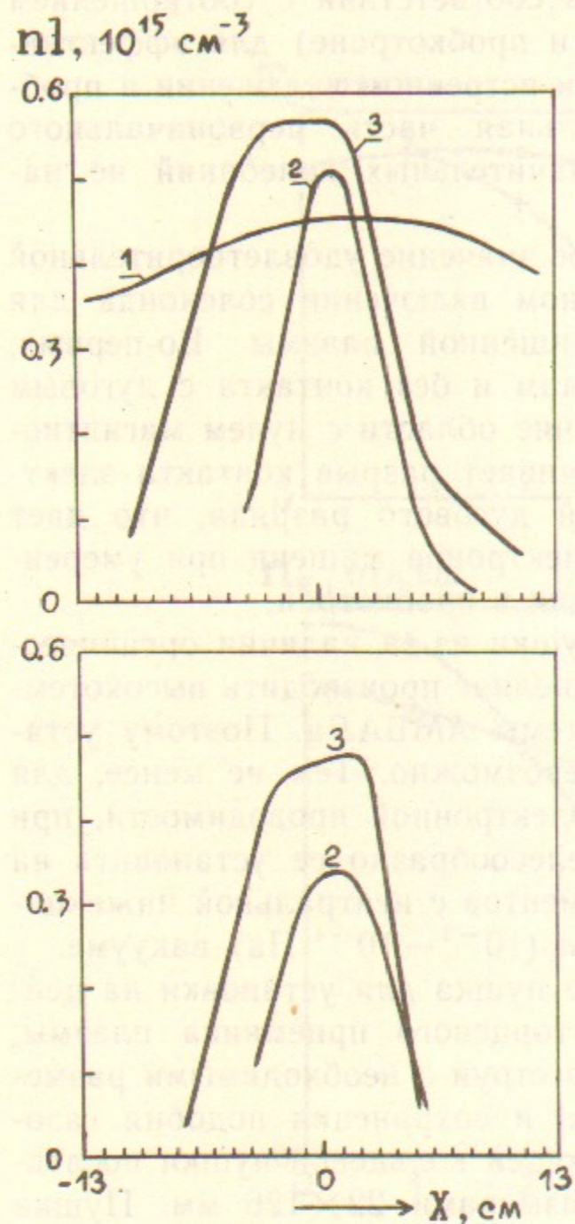
Рис. 25. Горизонтальный профиль линейной плотности плазмы осевой пушки, установленной в центральном фланце южного торцевого бака: a-l=1,75 м; b-l=2,25 м; 1—согласованное включение соленоида пушки, 2—соленоид выключен, 3—встречное включение.
