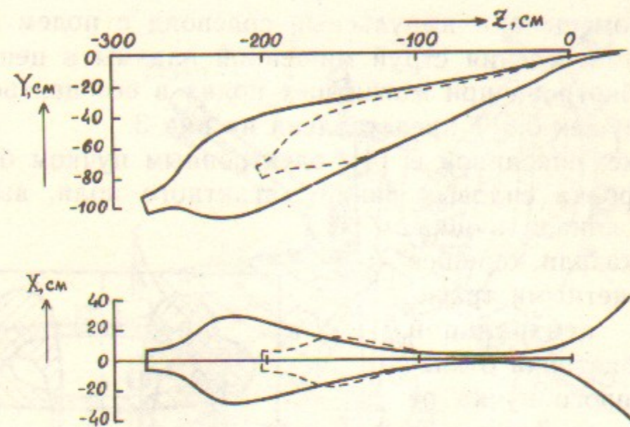
Рис. 4. Сечения силовой трубки магнитного поля, транспортирующей струю мишенной плазмы при l=2,95 м и l=2,15 м (штриховая линия): а — вертикальная плоскость; б — горизонтальная плоскость.
