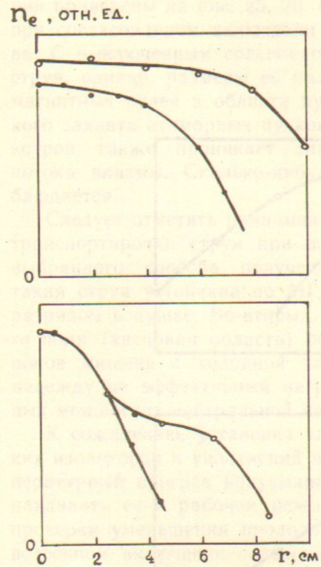
Рис. 22. Радиальное распределение плотности плазмы осевой пушки, (○ — согласованное включение соленоида пушки, ● — встречное включение): а — в сечении D; б — в сечении А.
