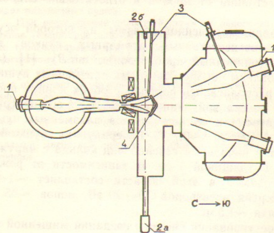
Рис. 2. Вертикальный разрез установки АМБАЛ-Ю:
