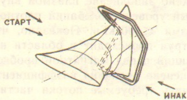
Рис. 6. Диамангнитная петля.
