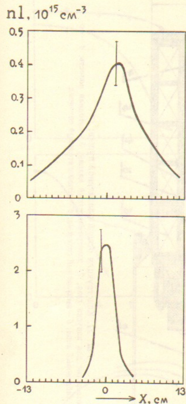
Рис. 19. Горизонтальный профиль линейной плотности плазменной струи пушки без соленоида, установленной в центральный фланец (а) — южного, (б) — северного торцевого приемного бака; l=1,75 м.
