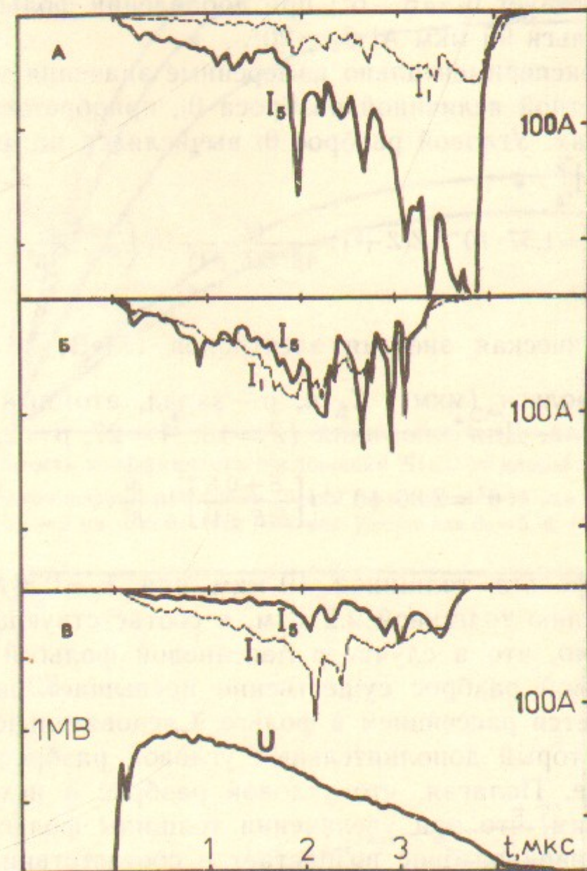
Рис. 5. Осциллограммы токов I_1 и I_5 при разной толщине анодной фольги.
