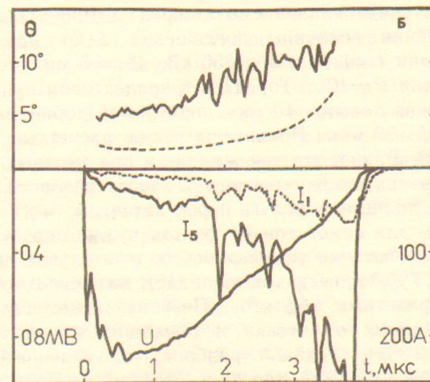
Рис. 8. Зависимость углового разброса от времени: а — лавсан + 90 мкм Al (№ 1008); б — лавсан 10 мкм (№ 1001); пунктиром — разброс в фольгах.
