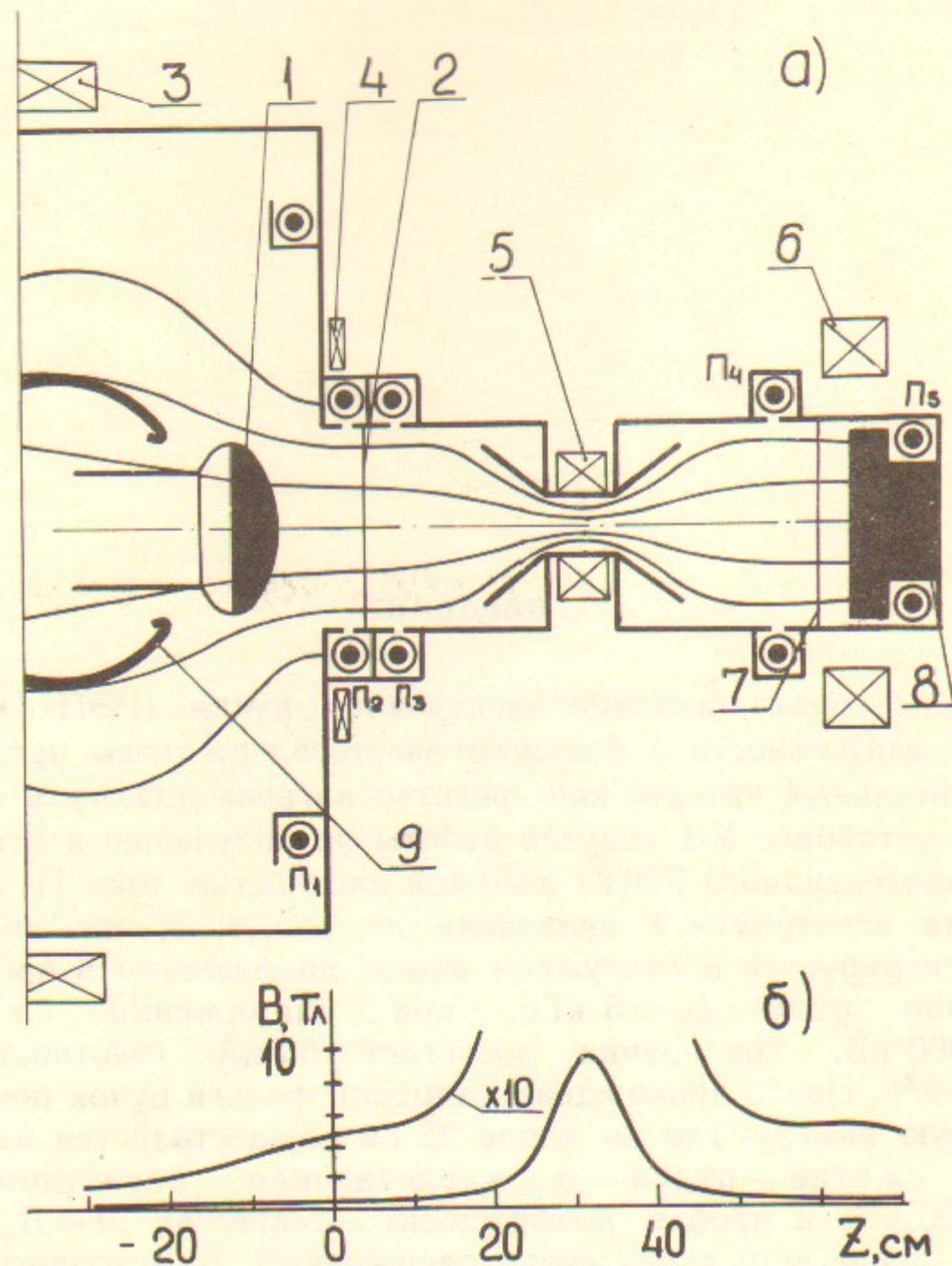
Рис. 1. Схема эксперимента по сжатию пучка:
