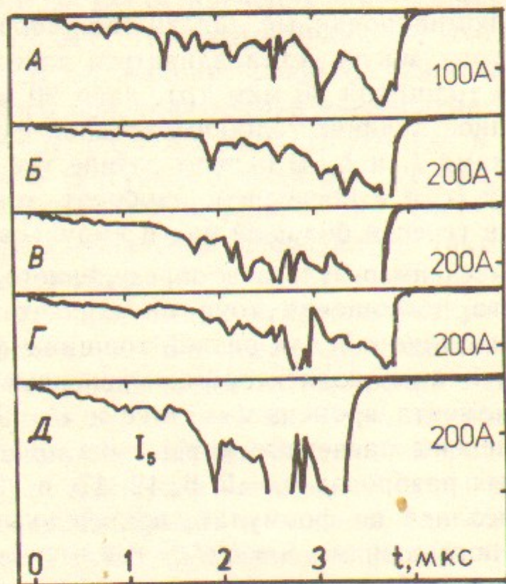
Рис. 4. Осциллограммы тока I_5 в разных выстрелах.
