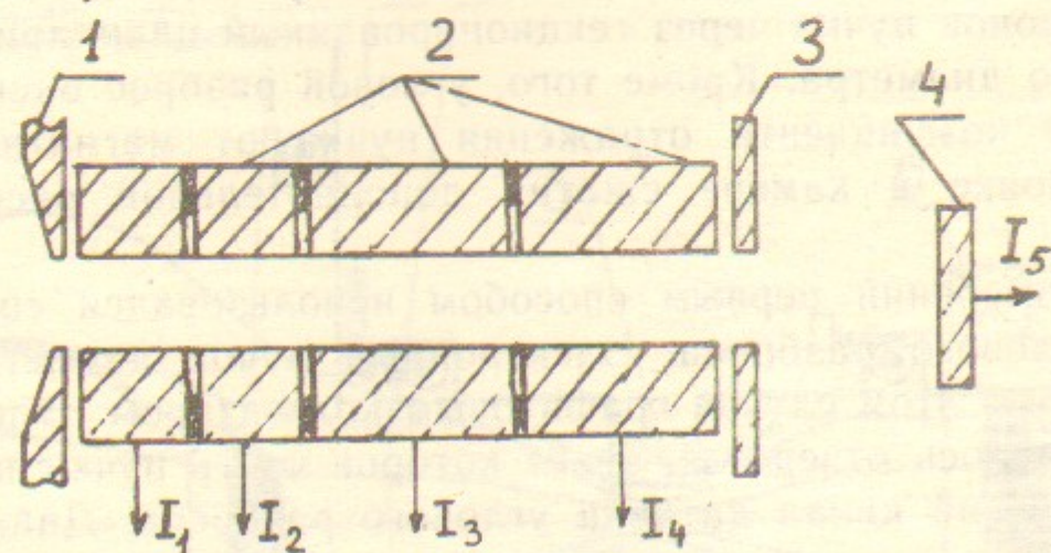
Рис. 2. Схема датчика углового разброса:
