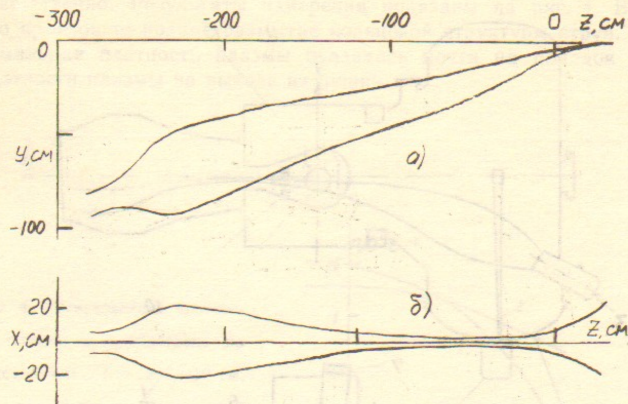
Рис. 2. Сечения силовой трубки магнитного поля, транспортирующего струю мишенной плазмы.
