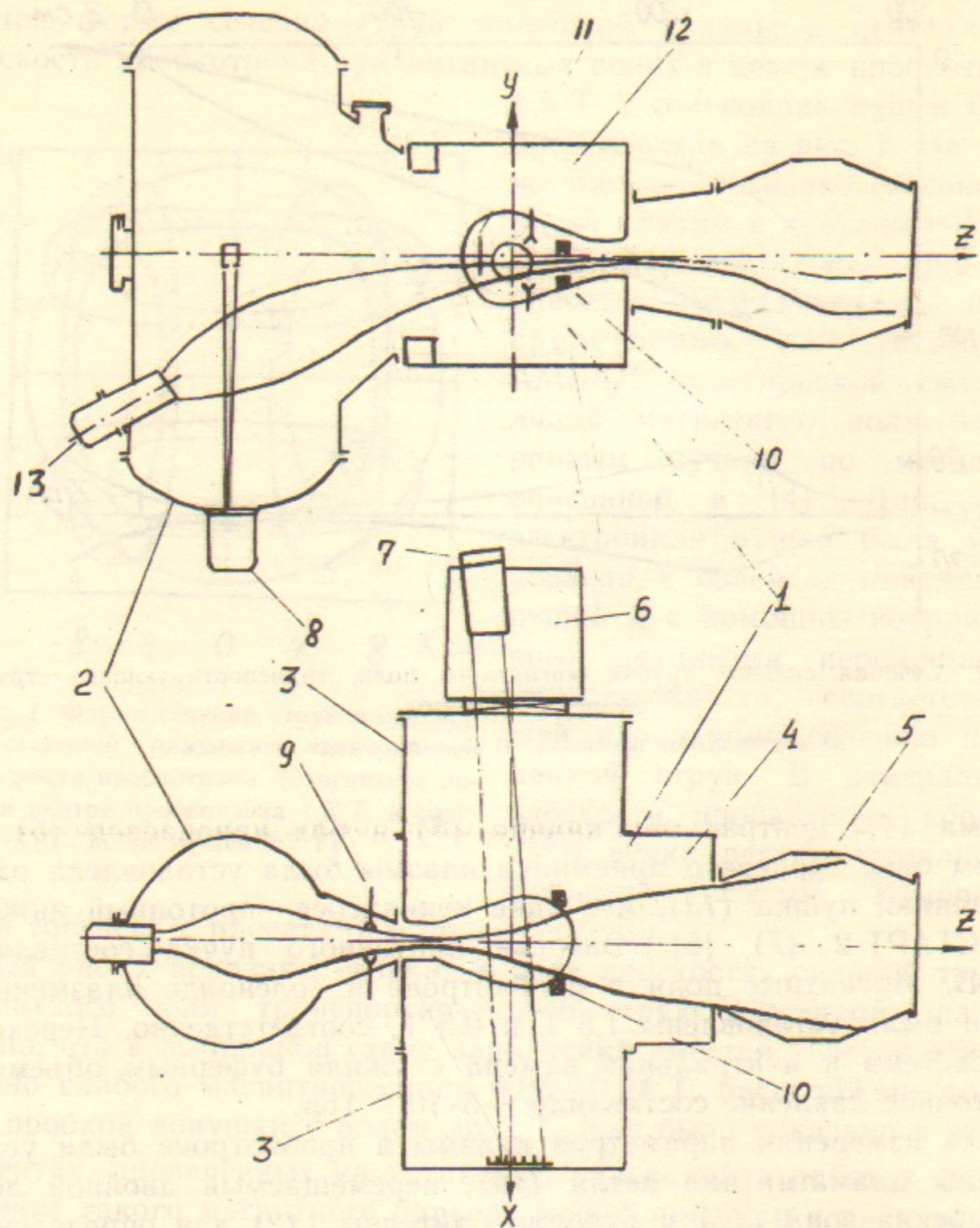
Рис. 3. Схема эксперимента.
