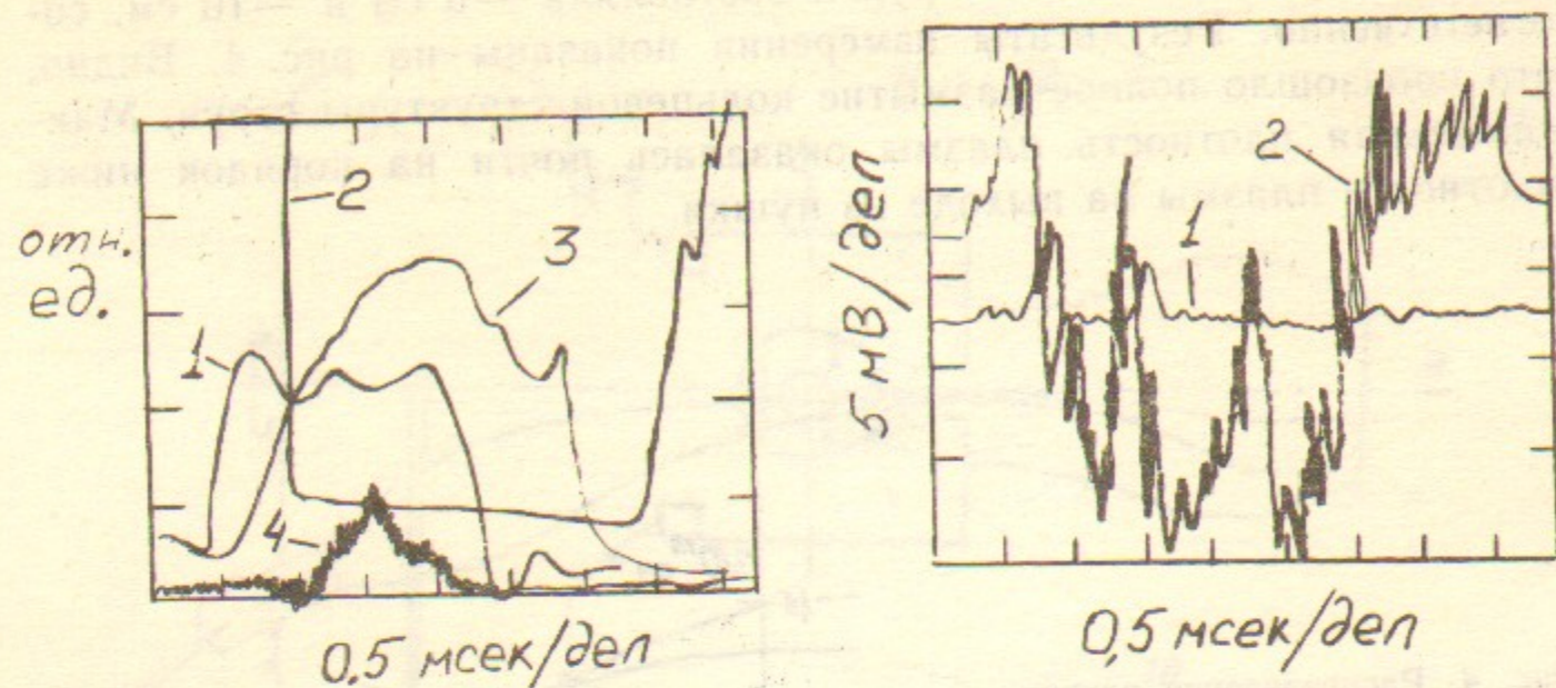
Рис. 6. Сигнал СВЧ-отсечки, \lambda=4 мм:
