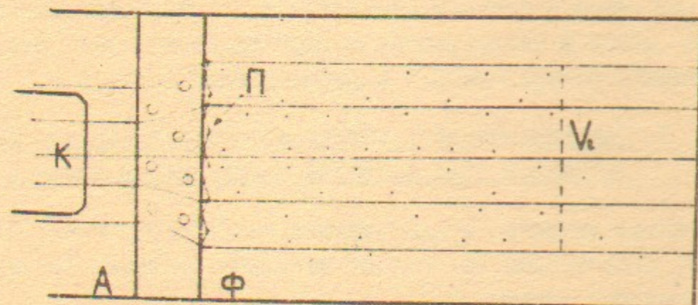
Рис.2. Ускорение ионов в неоднородном магнитном поле, К - катод, А - анодная фольга, Ф - фольга, разделяющая область ускорения и нейтрализующую плазму, кружки - объем, занятый нейтрализующей плазмой, точки - "синтезированная плазма", П - поверхностная плазма.
