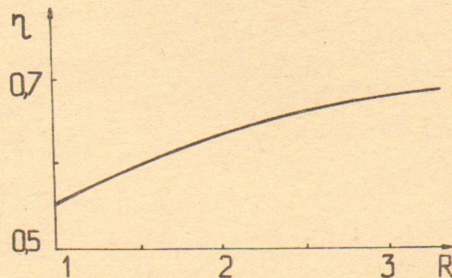
Рис. II. Зависимость КПД ускорения ионов от R .
