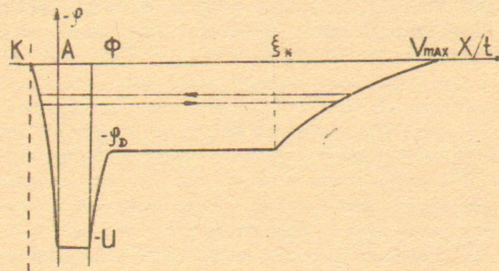
Рис.3. Форма потенциальной ямы для осциллирующих электронов.
