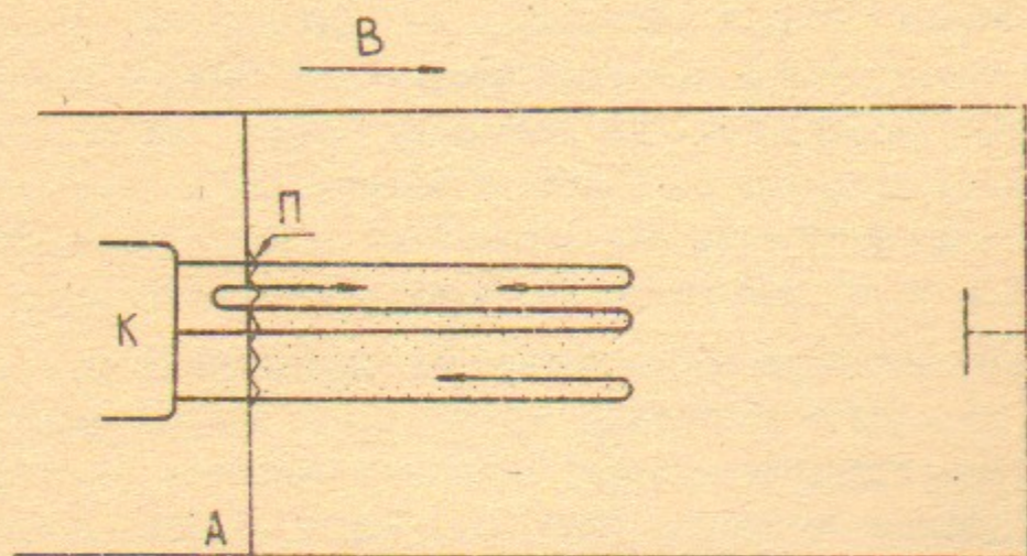
Рис.1. Схема газодинамического ускорения ионов: К - катод, А - анодная фольга, В - ведущее магнитное поле, П - поверхностная плазма, служащая источником ускоряемых ионов, точки - "синтезированная" плазма. Тонкие стрелки иллюстрируют характер движения электронов.
