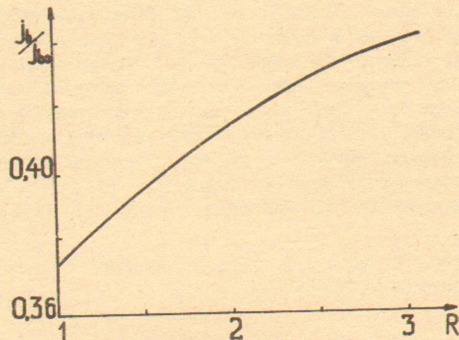
Рис. I0. Зависимость плотности диодного тока от уплотнения магнитного поля R .
