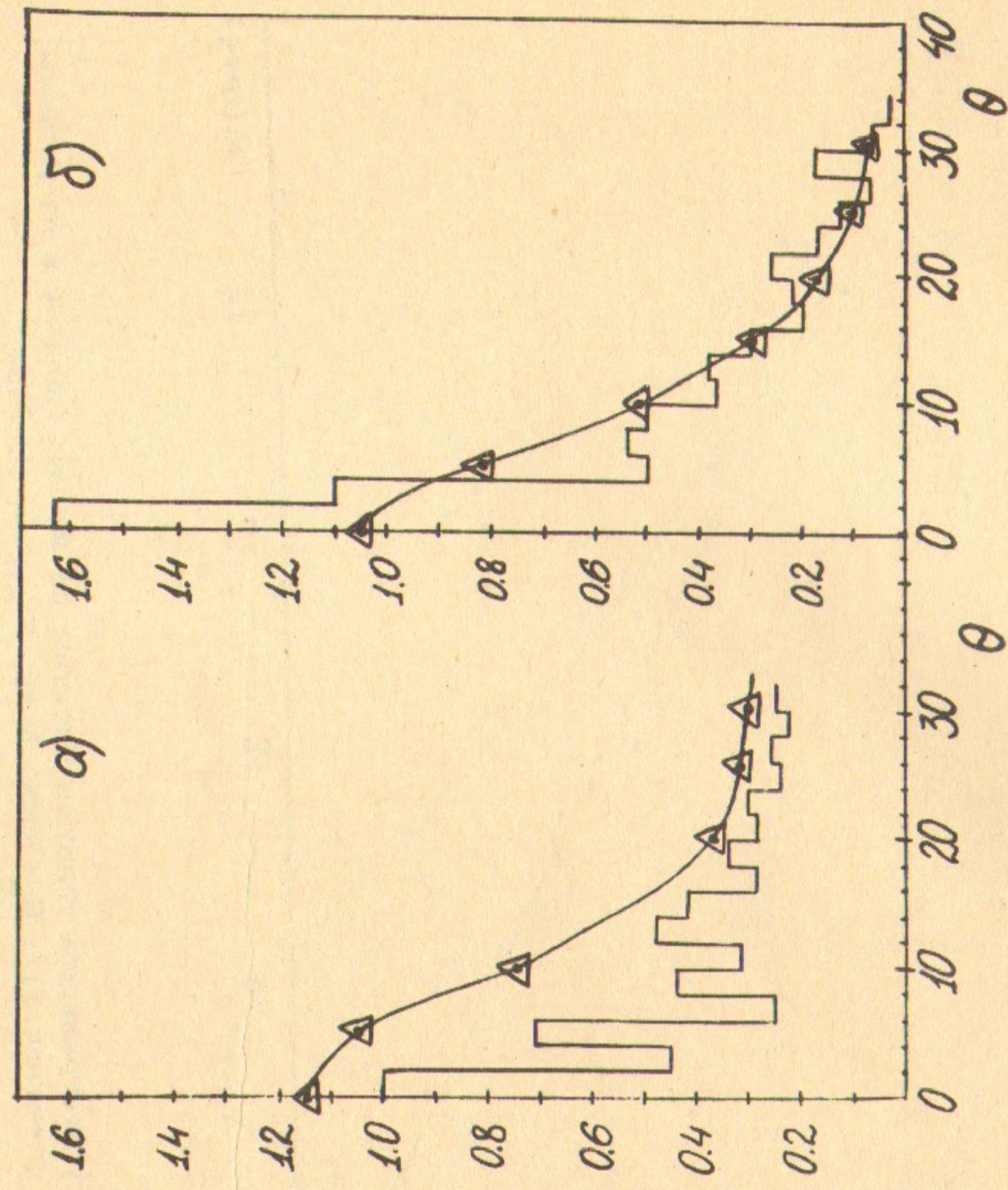
Рис. 10. Сравнение расчетных и экспериментальных угловых распределений в свинце: E_0 = 10000 Мэв; Z_M = 2,6 рад.дл.
